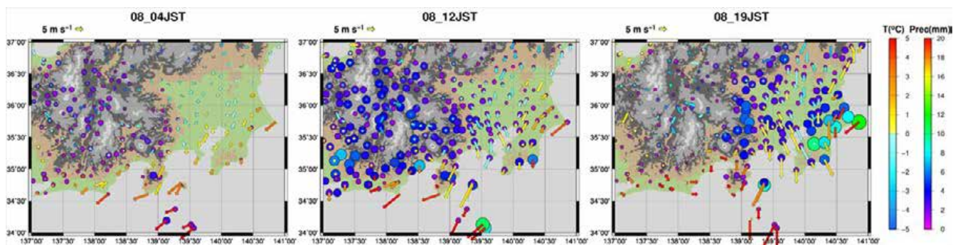
図1 case 08 の関東甲信地方の風向風速(矢印), 気温(矢印の色)及び降水量(●の色および大きさ)の分布. 日と時刻は各分布図の上を示す(JSTは日本標準時). 風について, 静穏(風力階級0, 0.3 \text{ ms}^{-1} 未満)は◇で表す.
