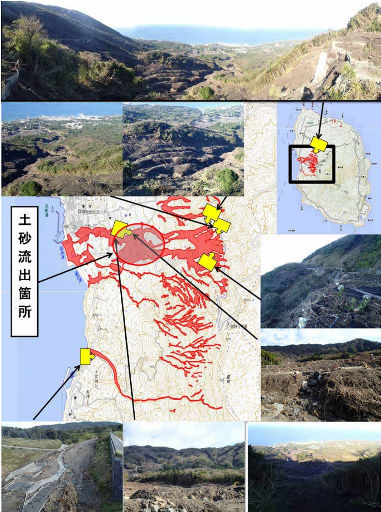
口絵 1 災害現場の状況（平成 25 年 11 月 13 ~ 14 日撮影），および土砂流出箇所（赤い塗りつぶし；データは国土地理院作成．背景地図は「地理院地図」（ http://maps.gsi.go.jp/ ）を利用）． Fig. 1 Photographs in Izu Oshima in 13 - 14 November 2013, and the distribution of debris flow (red area; data are produced by the Geospatial Information Authority of Japan). Background maps are the GSI Maps ( http://maps.gsi.go.jp/ ).
