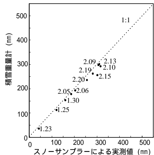
図 2 スノーサンプラーと積雪重量計で求めた積雪相当水量の関係
