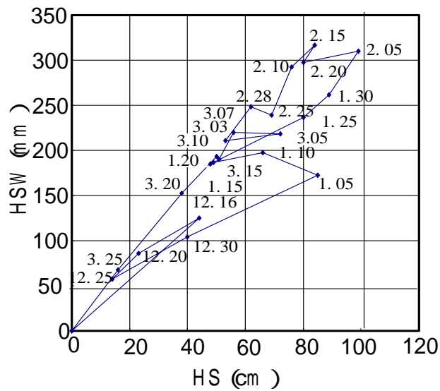
図 5 長岡雪氷研における積雪の深さと積雪の相当水量の循環曲線
