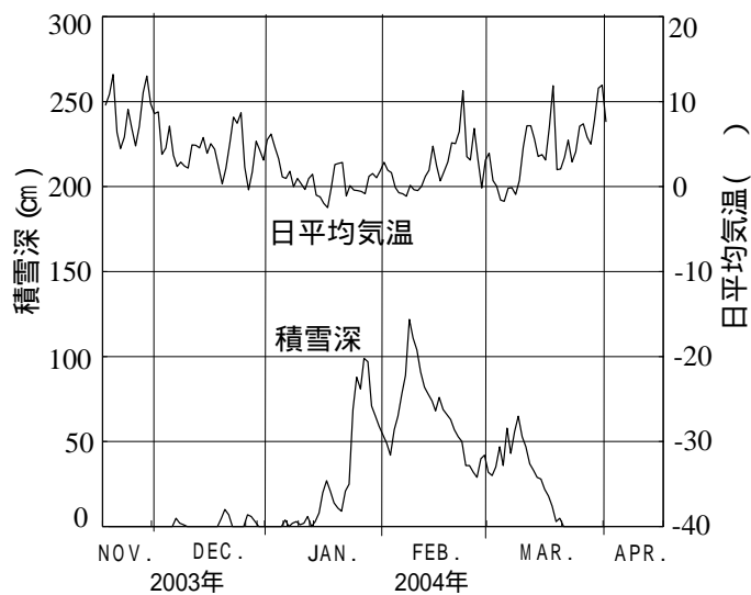
図3 長岡雪氷研における積雪深および日平均気温の時間変化 Fig. 3 Time series of the snow depth on the ground and daily mean temperature at NISIS.
