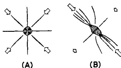
図10 火山下に働く圧力が等方な場合(A)とそうでない場合(B)の、割れ目発達の方の相違(Nakamura(1977)による)。
