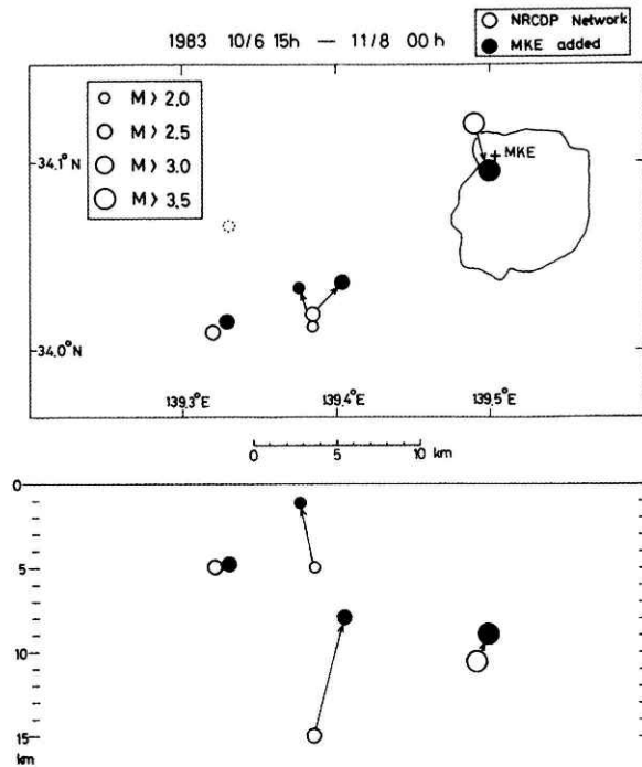
図13 既設観測網による震源位置と、現地データを加えて再決定された震源位置との比較
