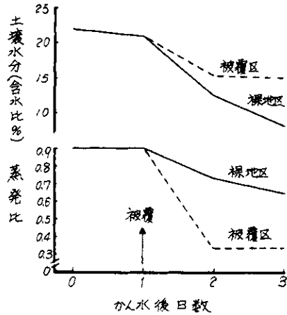
図7 発泡スチロール被覆による蒸発比 (Es/Ew)・土壤水分の経日推移
