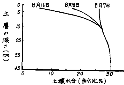
図4 深さ別土壌水分の経日変化
