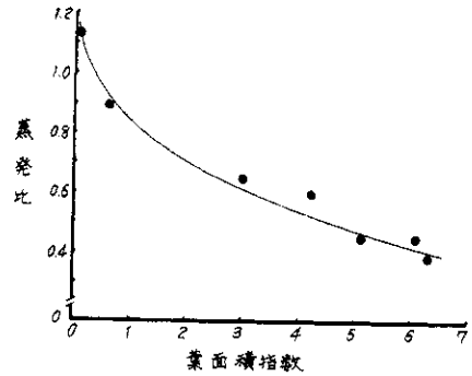
図5 トウモロコシ圃場における葉面積指数と蒸発比( E_s/E_w )との関係
