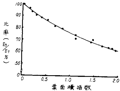
図6 ブドウ園における葉面積指数と土面蒸発量の蒸発数に対する比率( E_s/E_T %)との関係
