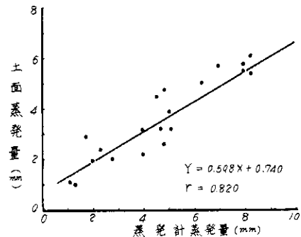
図2 モモ園における蒸発計蒸発量と土面蒸発量との関係
