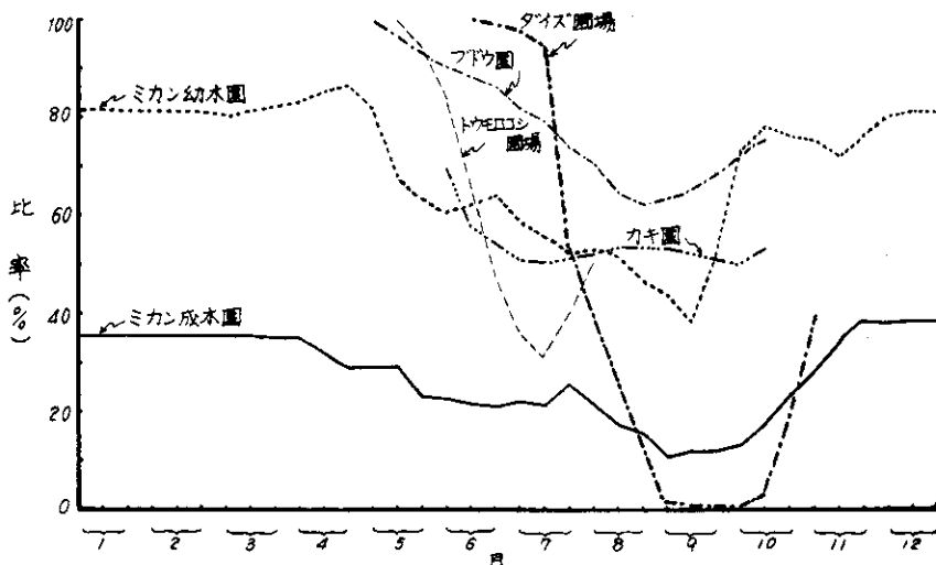
図1 蒸発散量に対する土面蒸発量の比率の生育時期別推移
