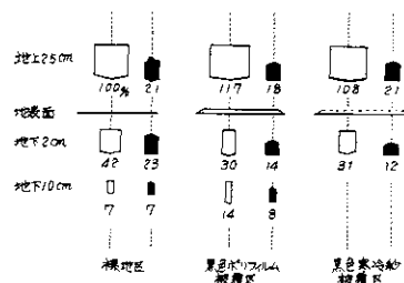
図9 被覆物の種類を異にした場合の地上・地中における熱流量(相対値)
