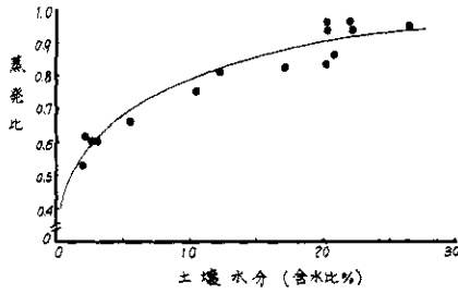
図3 土壌水分(含水比)と蒸発比( E_s/E_w )との関係
