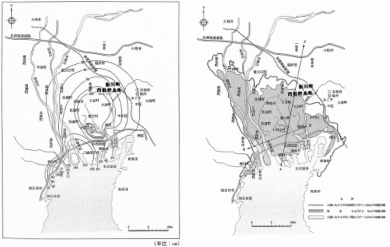
図 8 濃尾平野地盤沈下累積図：昭和 36 年から平成 8 年（愛知県，2000 を編集） Fig. 8 Total amount of ground subsidence from 1961 to 1998.
