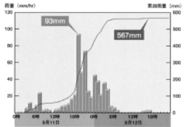
図3 2000 年東海水害時間雨量分布図（観測地点：名古屋地方気象台；国土交通省庄内川工事事務所，2000 を編集）
