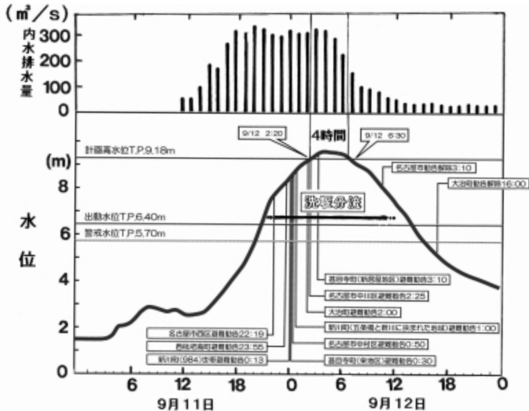
図 29 庄内川枇杷島地点の出水状況と内水排水ポンプ運転状況（国土交通省庄内川工事事務所（2000）を編集）
