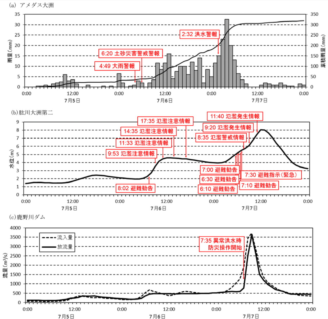
図 12 (a) アメダス大洲における 1 時間雨量と積算雨量, (b) 大洲第二観測所における肱川の水位, (c) 鹿野川ダムにおける流入量と放流量. 赤字は気象庁や大洲市からの防災情報
