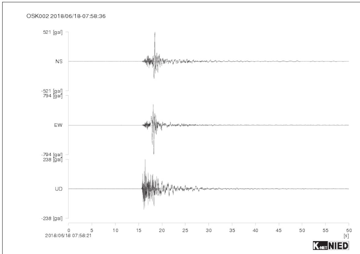
口絵 2 K-NET 高槻 (OSK002) 観測点の強震動波形 (K-NET・KiK-net)
