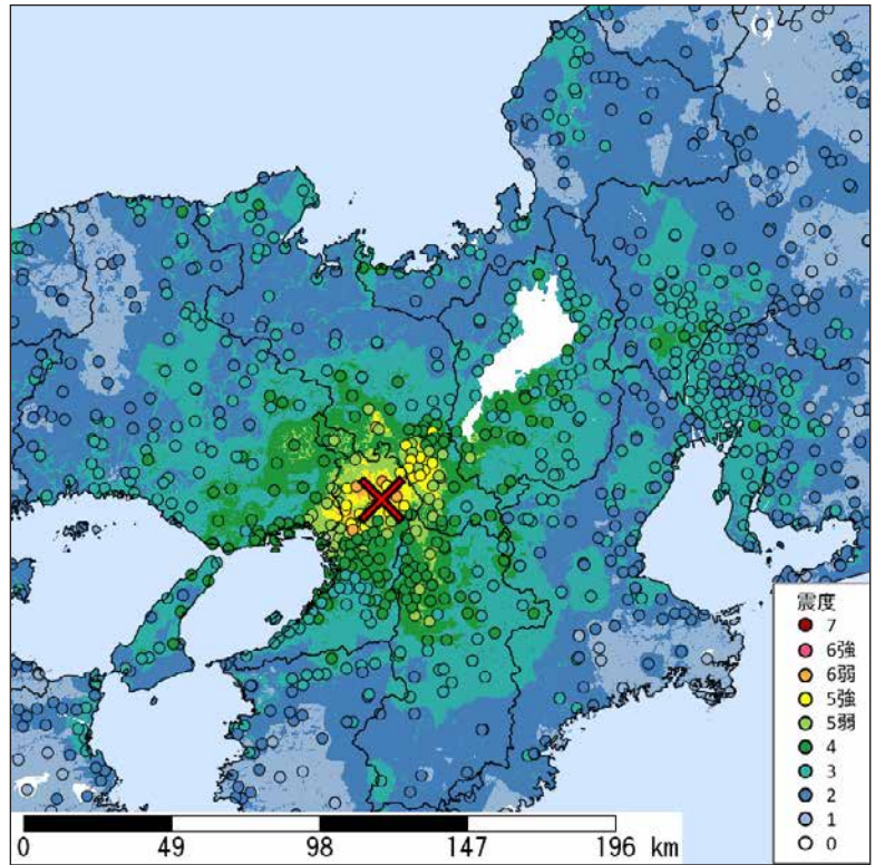
口絵 1 大阪北部の地震(2018年6月18日7時58分発生, M5.9)の震度分布 (J-RISQ 2018/06/18 08:10:35 発表 Ver.7 最終報)
