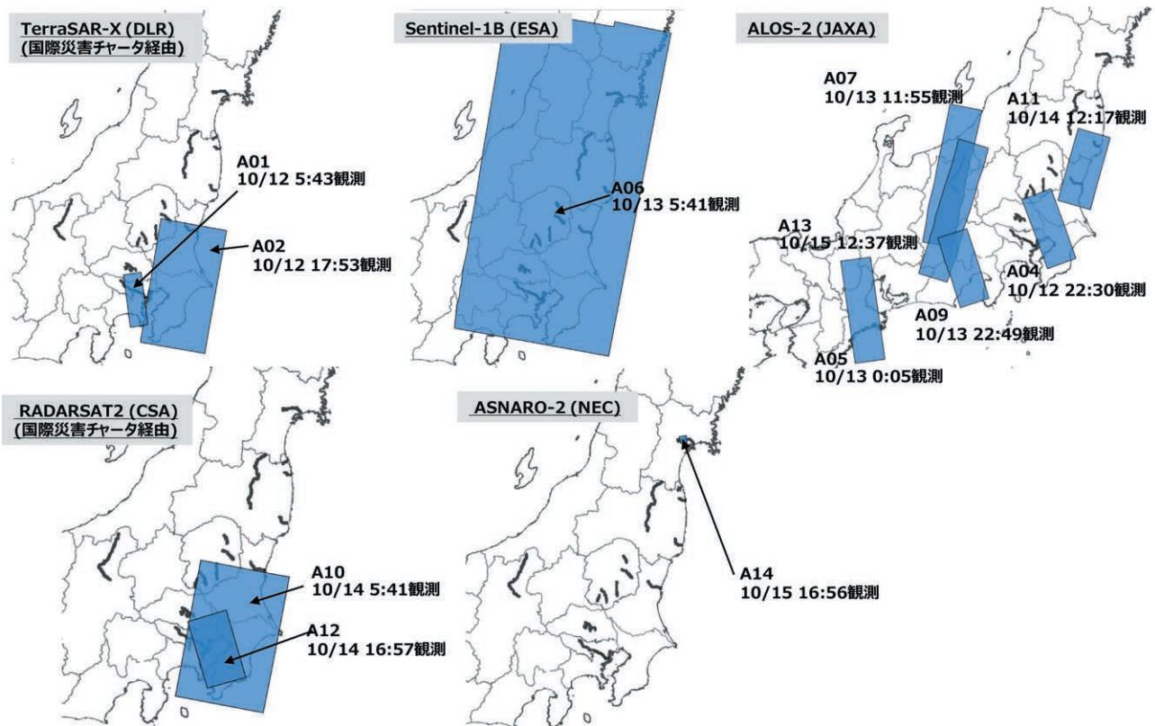
図 6 レーダ衛星の観測範囲
