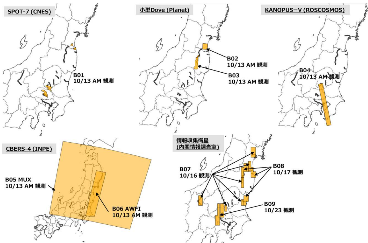
図 7 光学衛星の観測範囲
