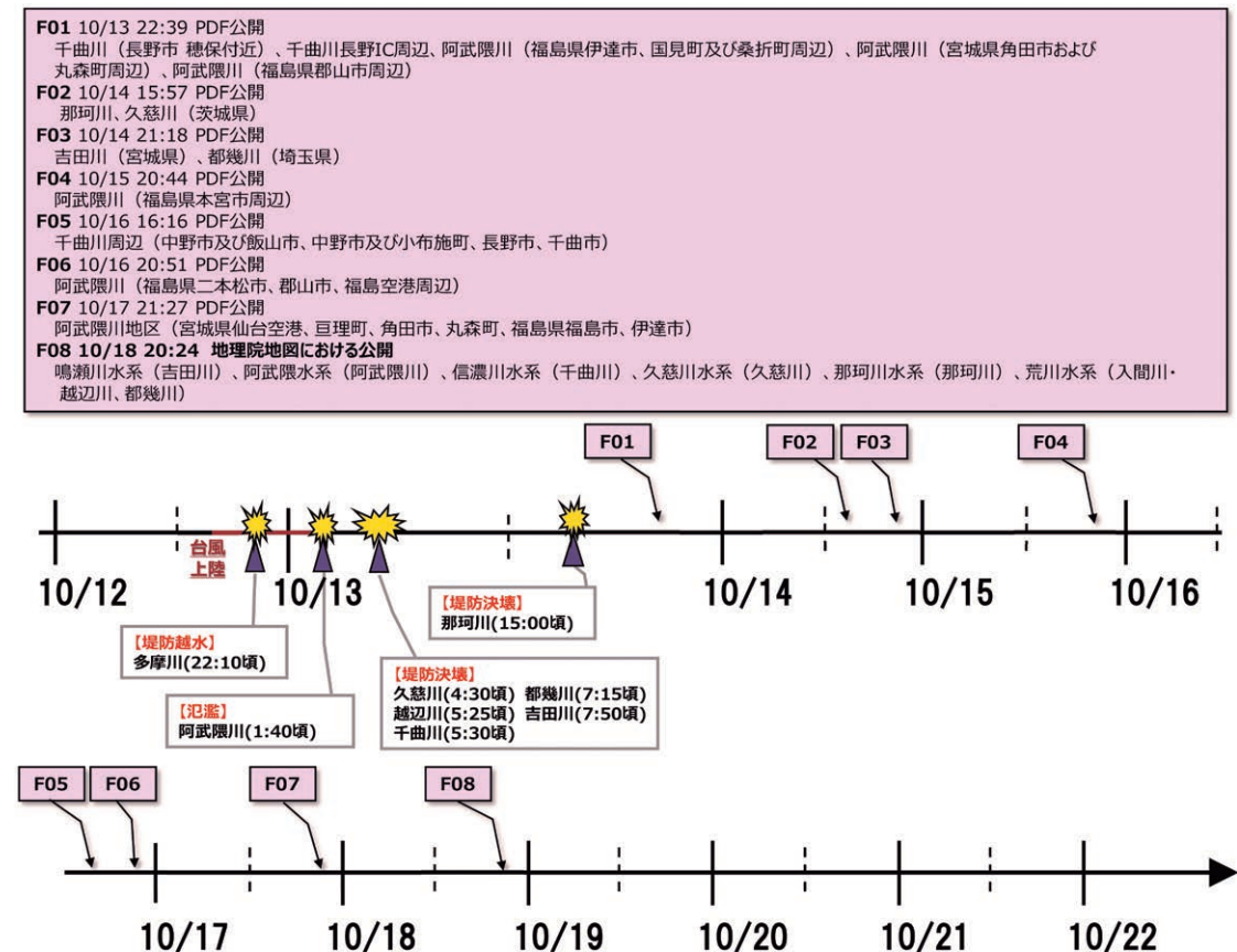
図5 国土地理院 浸水推定段彩図の公開タイミング
