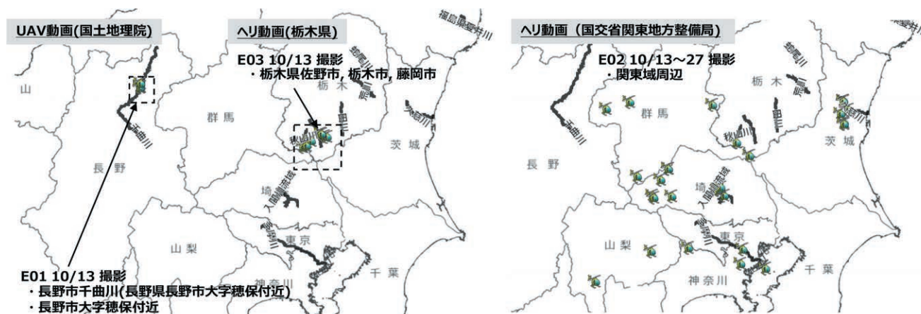
図11 ヘリ・UAV 動画の撮影地点
