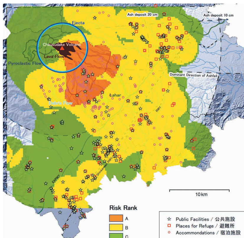
図 6 那須岳周辺地域の火山災害リスク評価結果 評価結果から高位から低位に A, B, C 地域に区分して図示. 火山災害リスク評価の結果から GIS で作成. 噴出物想定分布域は那須岳火山防災マップ(2010)から参照した.
