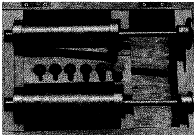
写真1 カナディアンハードネスゲージ(積雪硬度計)
