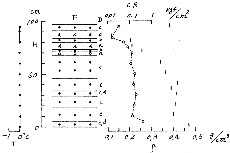
図3 積雪断面観測図(長岡)
