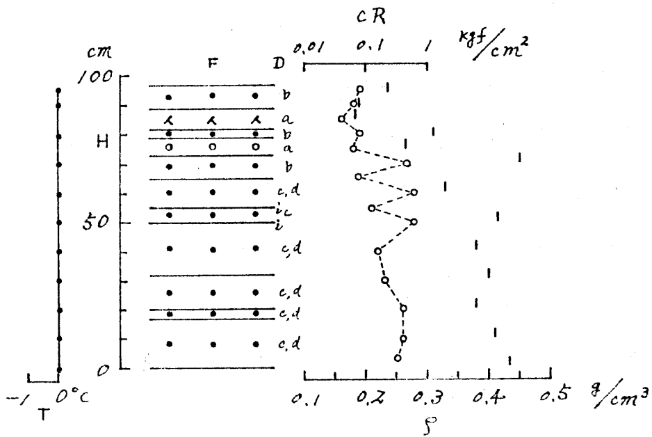
図 3 積雪断面観測図 (長岡)
