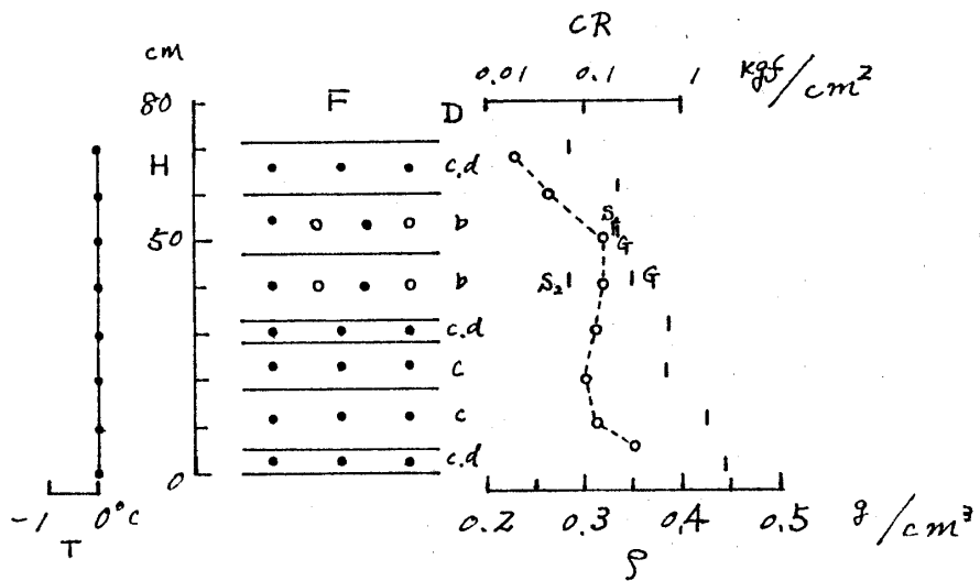
図3 積雪断面観測図(長岡)
