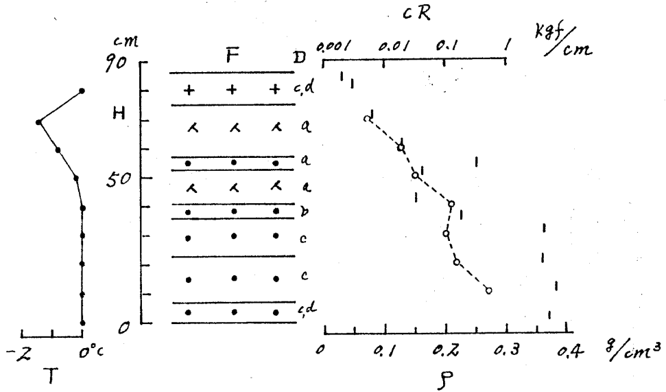
図3 積雪断面観測図(長岡)
