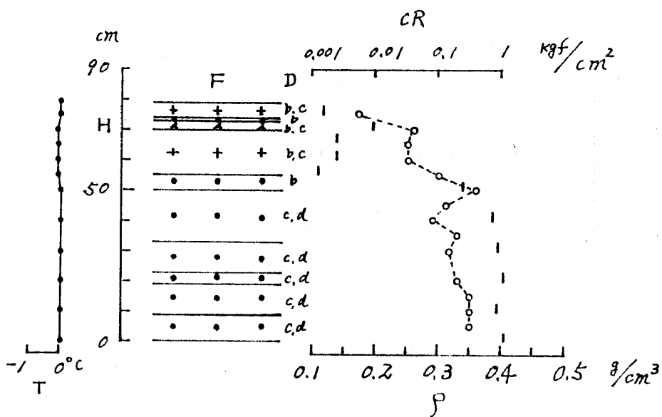
図3 積雪断面観測図(長岡)
