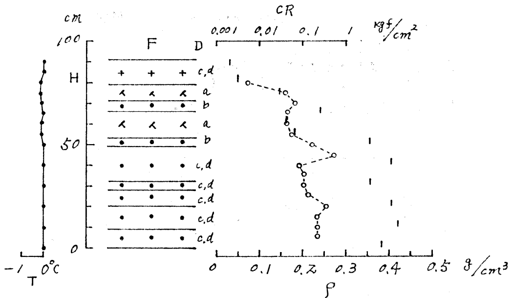
図3 積雪断面観測図(長岡)
