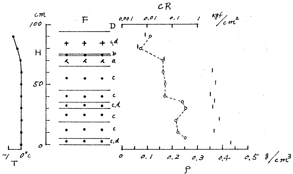
図3 積雪断面観測図(長岡)
