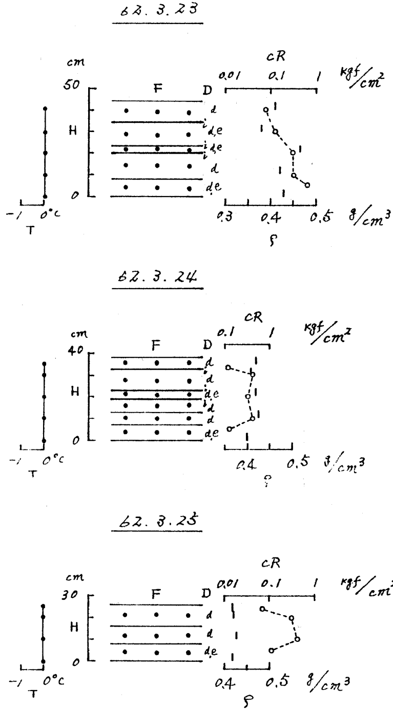
图3 积雪断面観測図(長岡)
