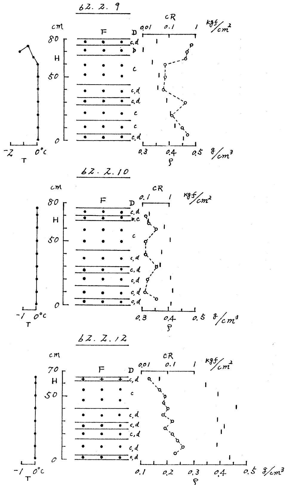
図3 積雪断面観測図(長岡)
