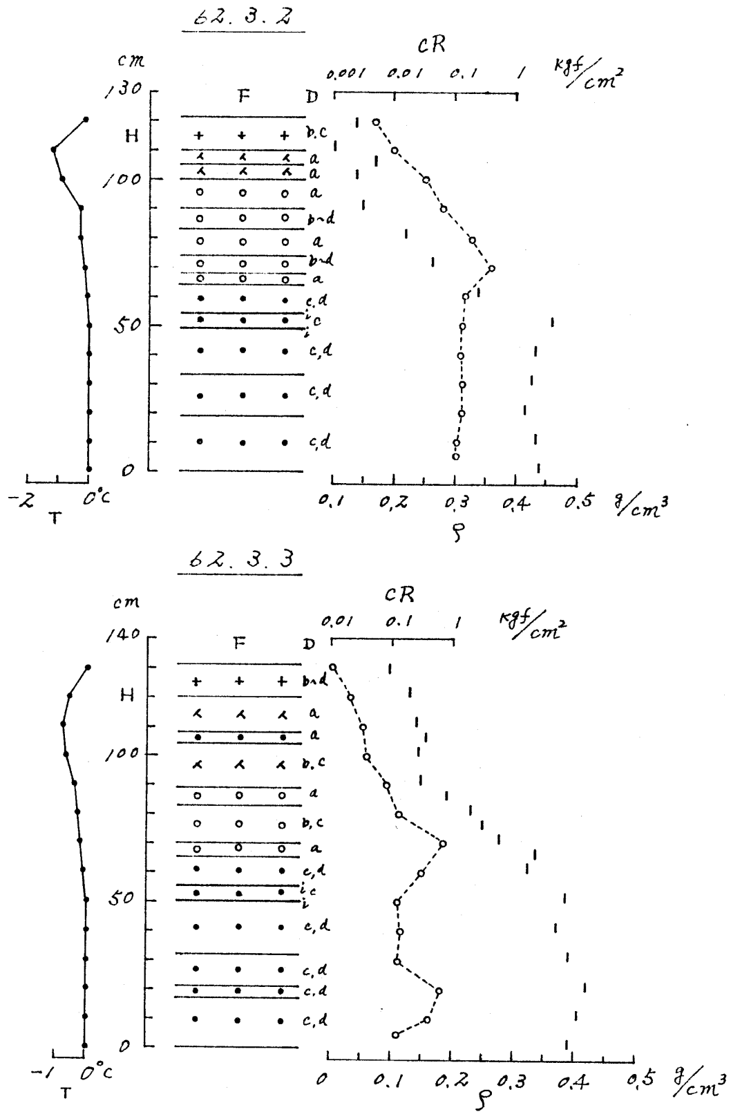
図3 積雪断面観測図(長岡)
