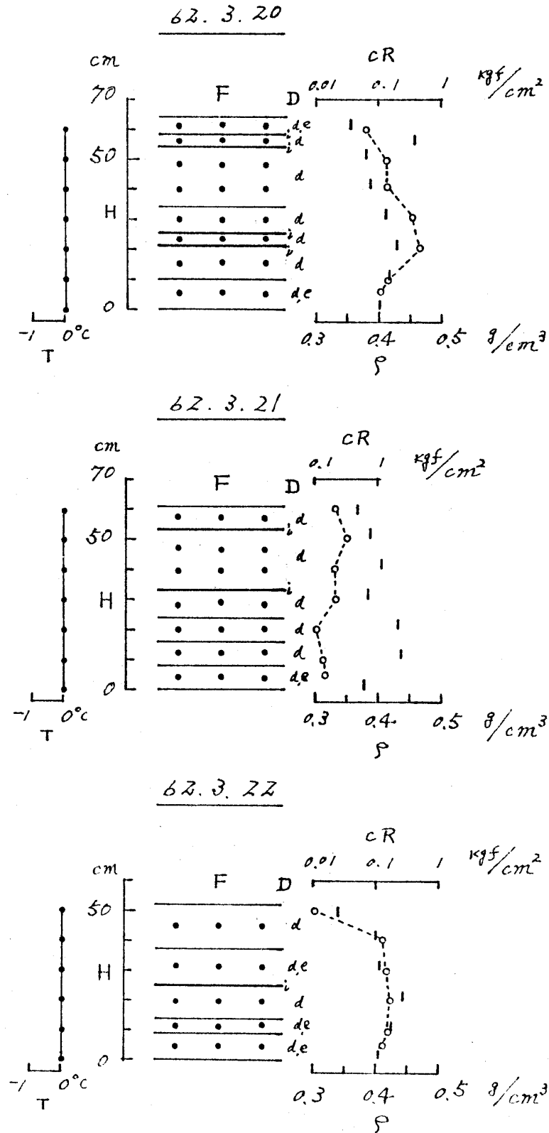
図3 積雪断面観測図(長岡)
