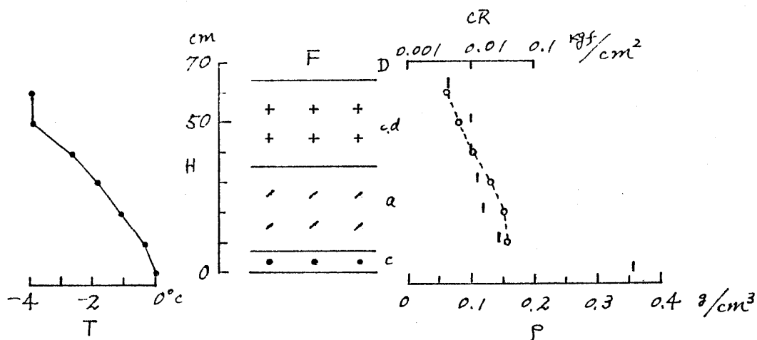
図3 積雪断面観測図(長岡)
