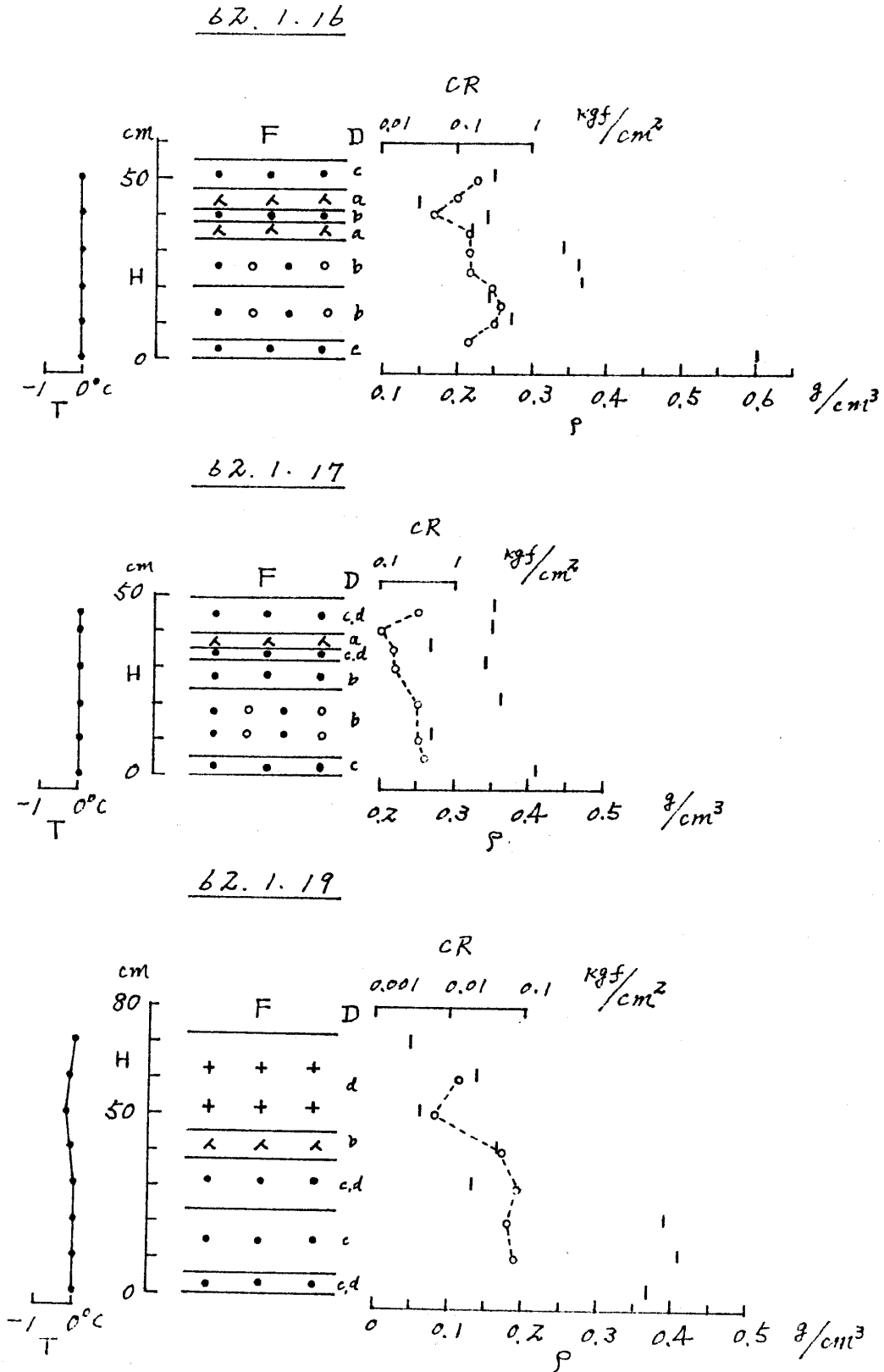
図3 積雪断面観測図(長岡)
