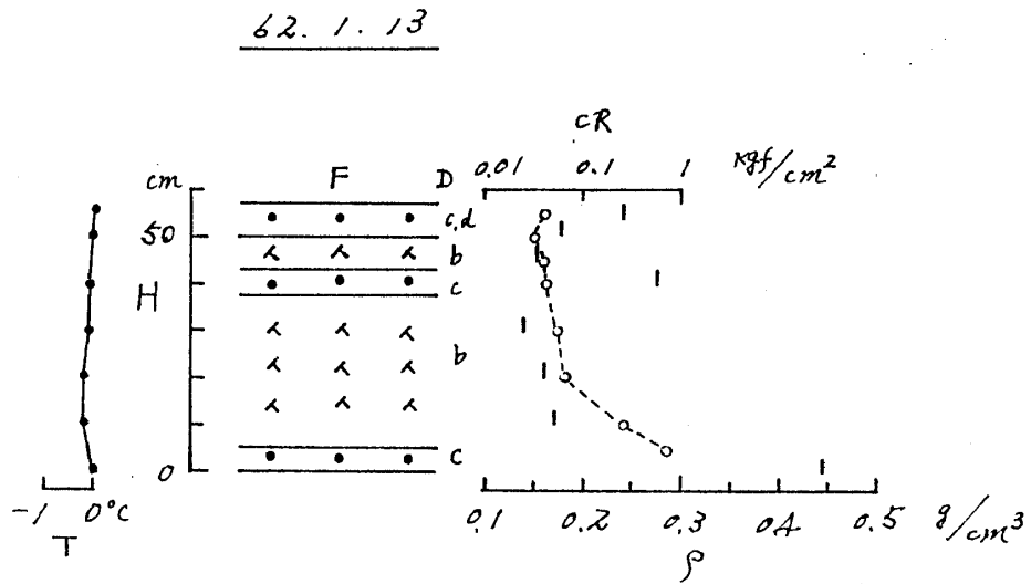
図3 積雪断面観測図(長岡)
