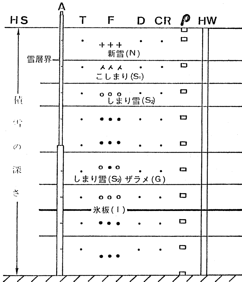
図2 積雪断面観測の観測項目と測定位置
