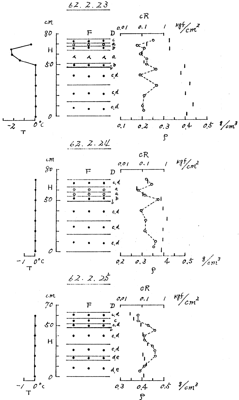
图3 积雪断面観測図(長岡)
