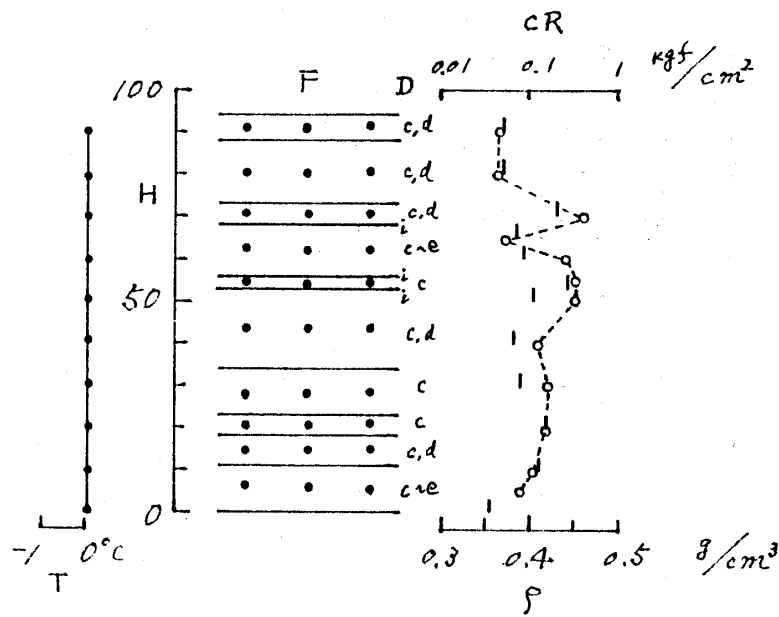
図3 積雪断面観測図(長岡)
