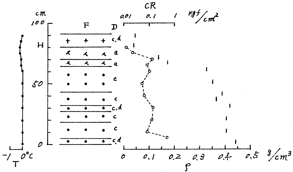
图3 积雪断面観測図(長岡)
