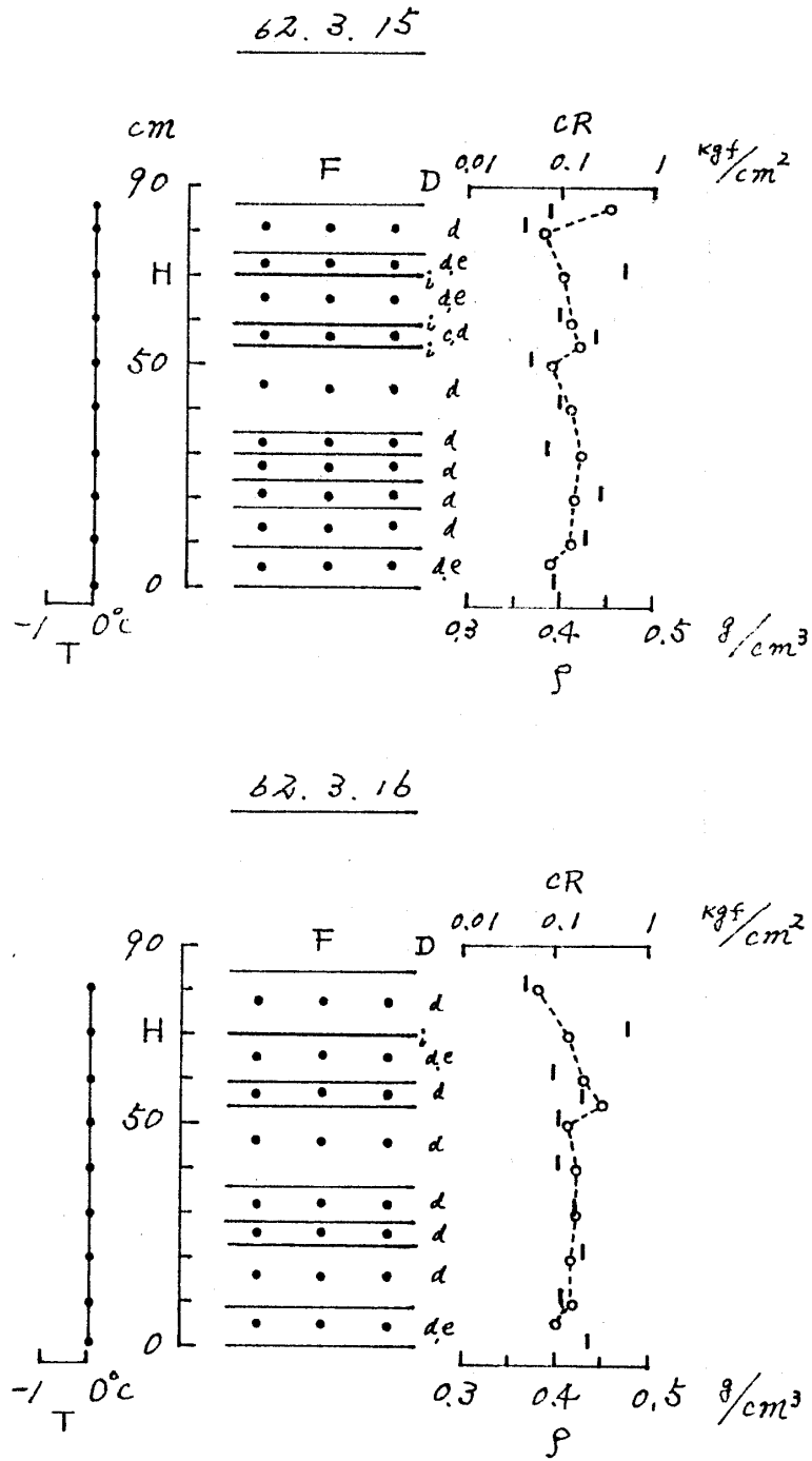
図3 積雪断面観測図(長岡)
