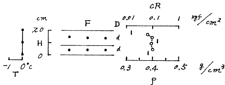
図3 積雪断面観測図(長岡)
