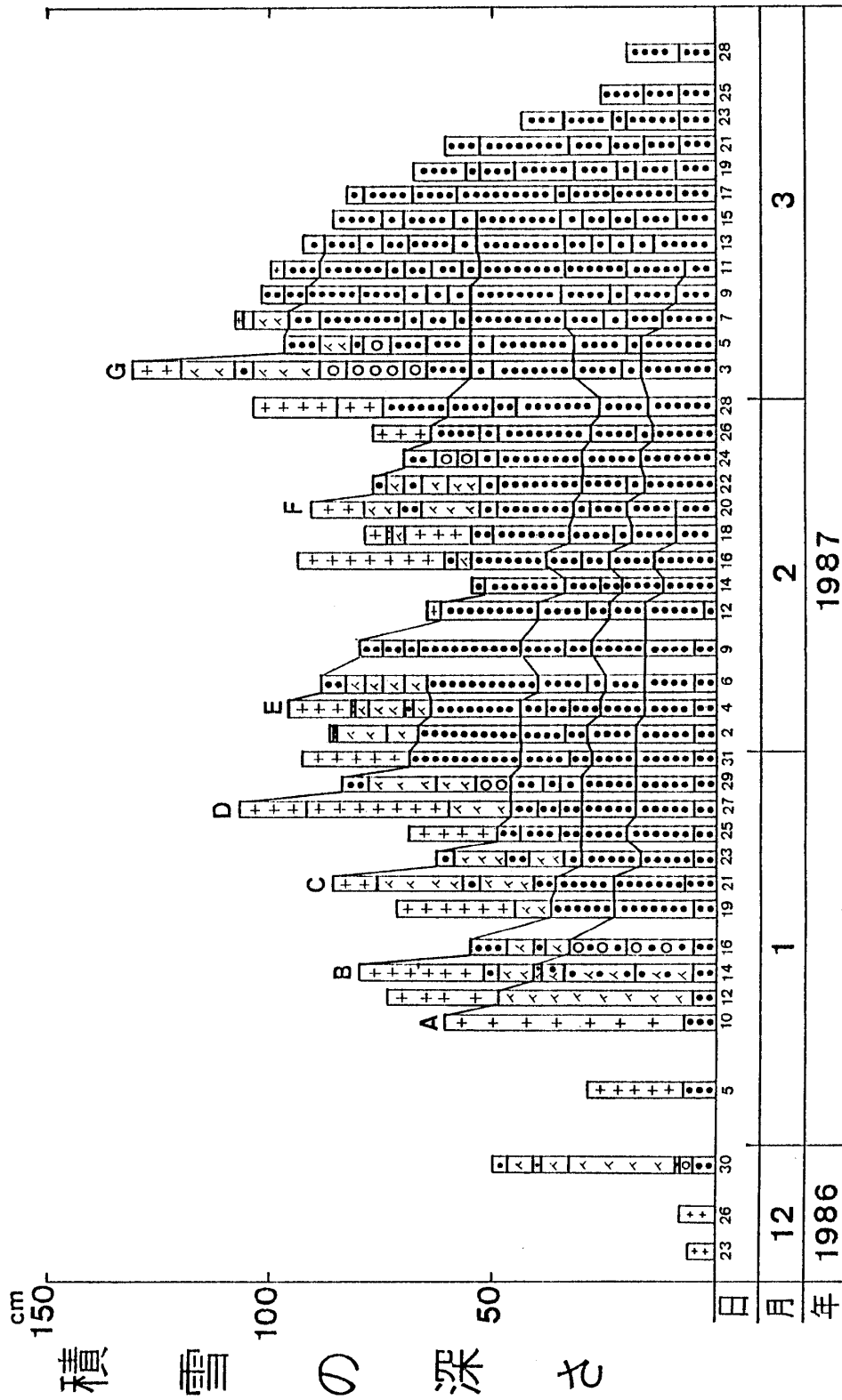
図5 積雪層の経時変化
