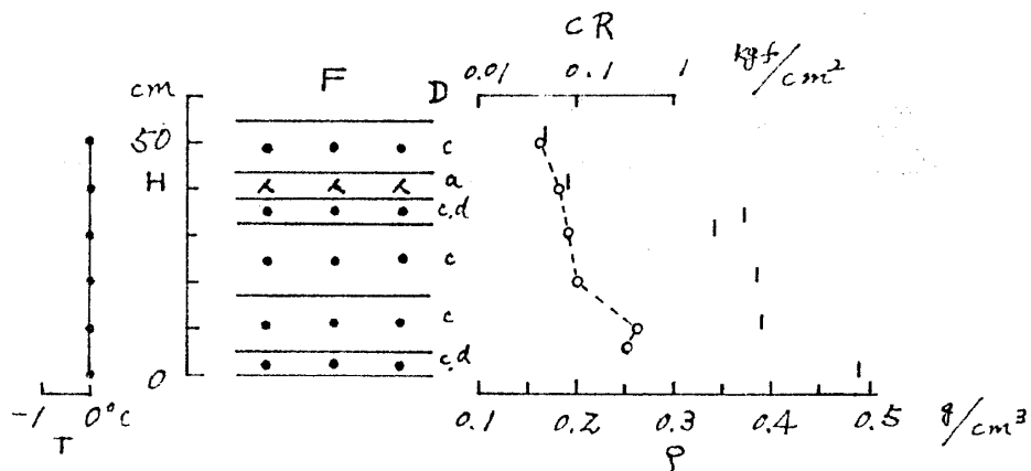
図3 積雪断面観測図(長岡)
