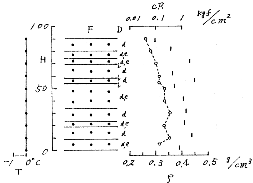
図3 積雪断面観測図(長岡)
