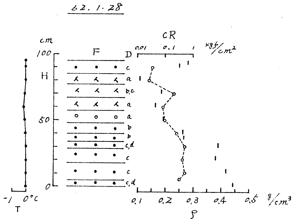
図3 積雪断面観測図(長岡)
