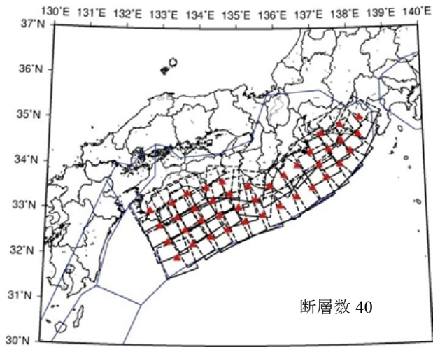
図 2.4.4.3-10 南海トラフ沿いの M \geq 7.6 の地震の断層面 (▲: 断層中心, プレート間地震の断層面はプレート上面に沿うように, プレート内地震の断層面はそれよりも 10km 深いところに配置)
