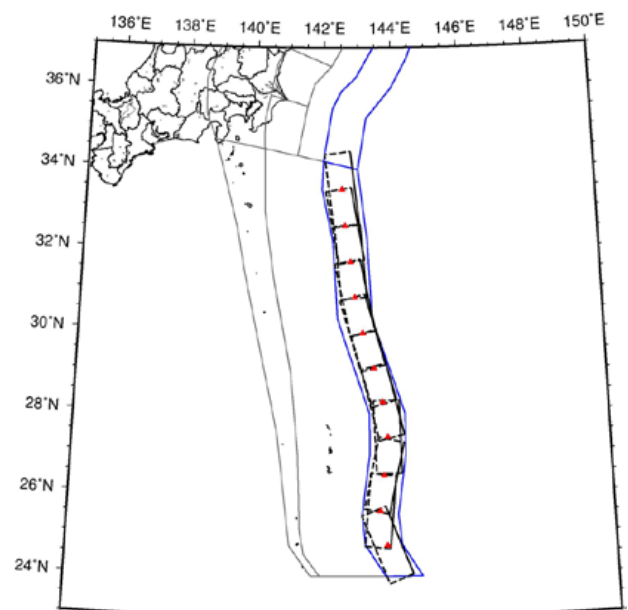
M8.1～M8.2 (200km×100km)
