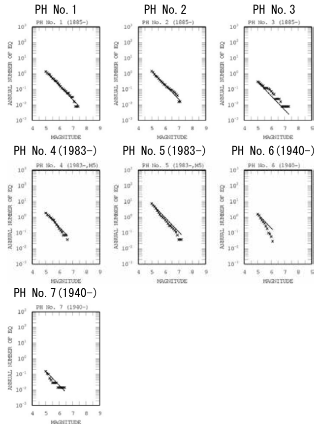
図 2.4.4.3-4 中地震カタログに基づく地震の規模別累積頻度
