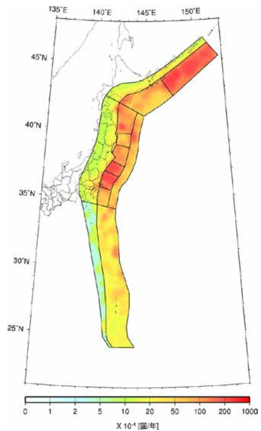
図 2.4.3.3-10 太平洋プレートの地震の発生頻度 (0.1 度四方あたり, M5.0 以上)
