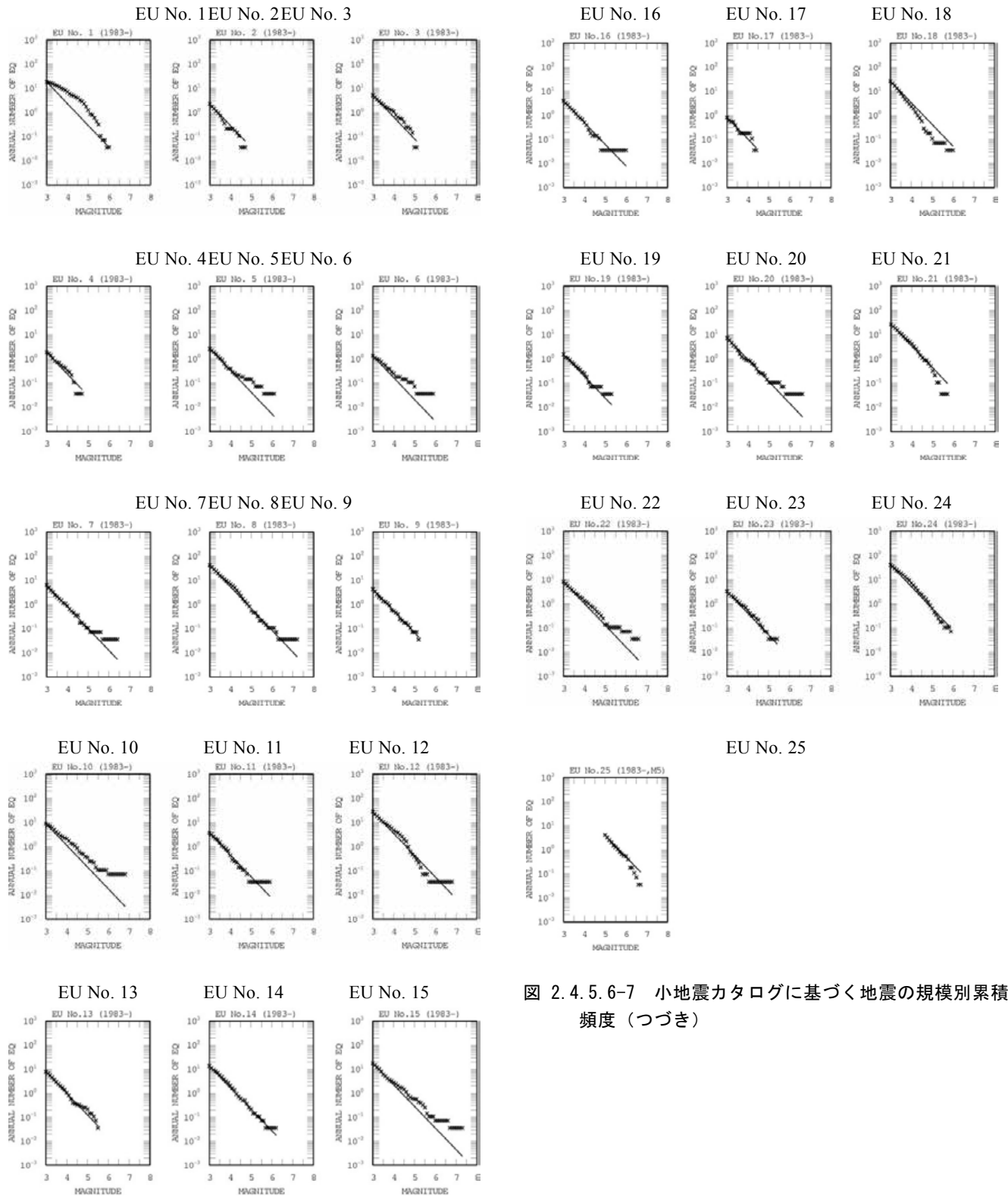
図 2.4.5.6-7 小地震カタログに基づく地震の規模別累積 頻度
