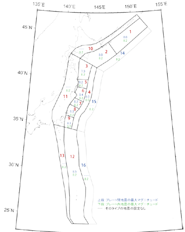
図 2.4.3.3-7 領域ごとの地震の最大マグニチュード
