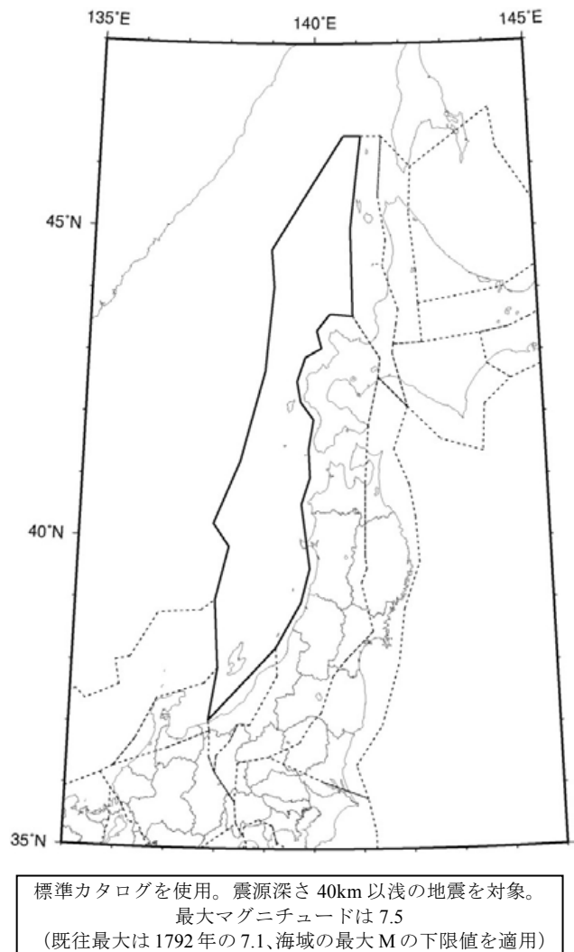
図 2.4.5.6-14 日本海東縁部の震源断層を予め特定しにくい地震の地域区分、使用する地震カタログ、および最大マグニチュード。（陸域の浅い地震の地域区分も点線で表示）
