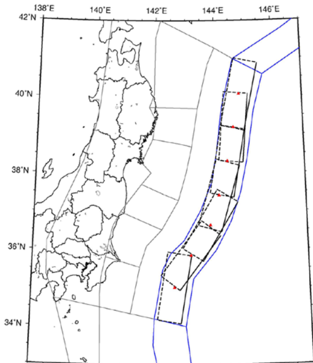
M8.1～M8.2 (200km×100km)
