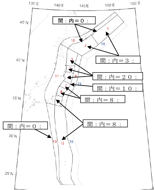
図 2.4.3.3-9 領域ごとのプレート間地震とプレート内地震の比
