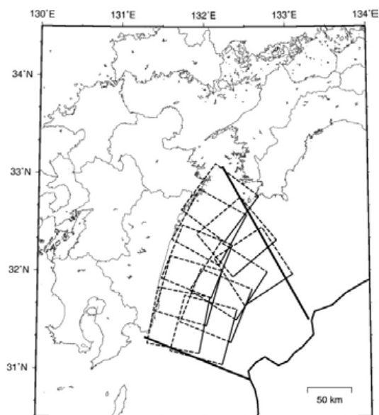
図 2.4.4.2-1 日向灘のプレート間地震の断層面
