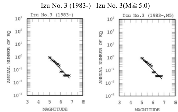
図 2.4.5.6-24 伊豆諸島以南の震源断層を予め特定しにくい地震の規模別累積発生頻度（左：中地震カタログ，右：小地震カタログ）
