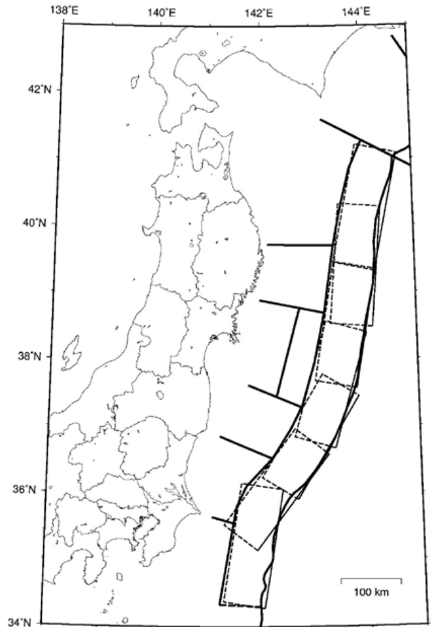
図 2.4.3.2-2 三陸沖北部から房総沖の海溝寄りのプレート内大地震 (正断層型) の断層面
