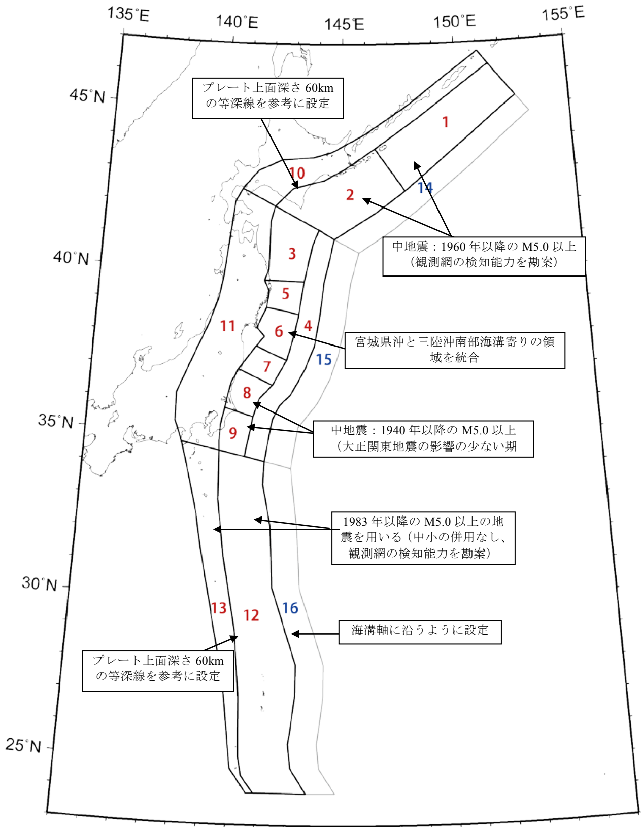
図 2.4.3.3-2 太平洋プレートの震源断層を予め特定しにくい地震の地域区分と頻度算定に用いる地震カタログ。特記のない場合は、標準カタログを使用。海溝軸の外側の 3 領域（青字）は後述のアウトターライズの地震の領域。
