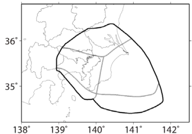
図 2.4.4.1-1 相模トラフ沿いの M8 クラスの地震の対象領域。黒い太線が最大クラスの地震の想定震源域、灰色の線は領域を分割する際に参照する線で、東西方向の 2 本はプレート上面深さ 10km と 30 km の等深線、南北方向は大正型関東地震の震源域のほぼ東端。
