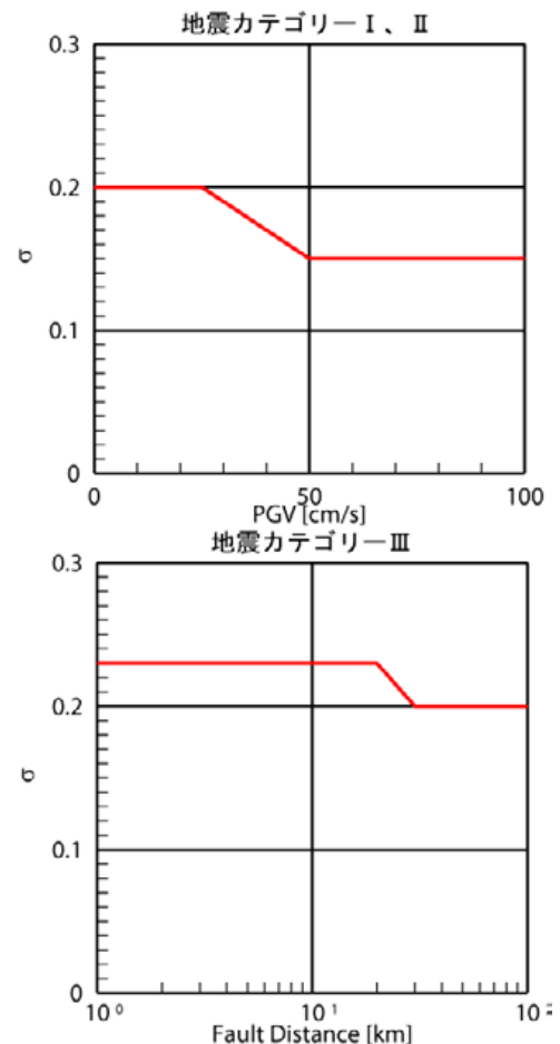
図 2.6.3-1 地震動評価に適用するばらつき ( \sigma ; 常用対数標準偏差) の値 (赤線)
