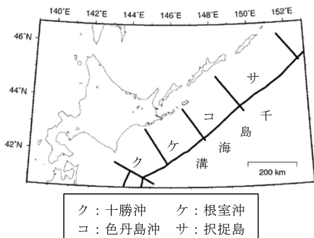
図 2.4.3.1-1 千島海溝沿いの海溝型地震の評価対象領域
