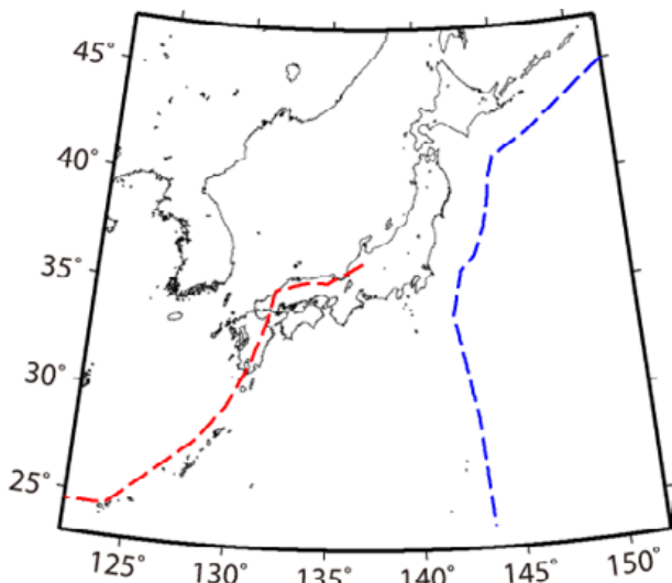
図 2.6.2-1 海溝軸（青）と火山フロント（赤）
