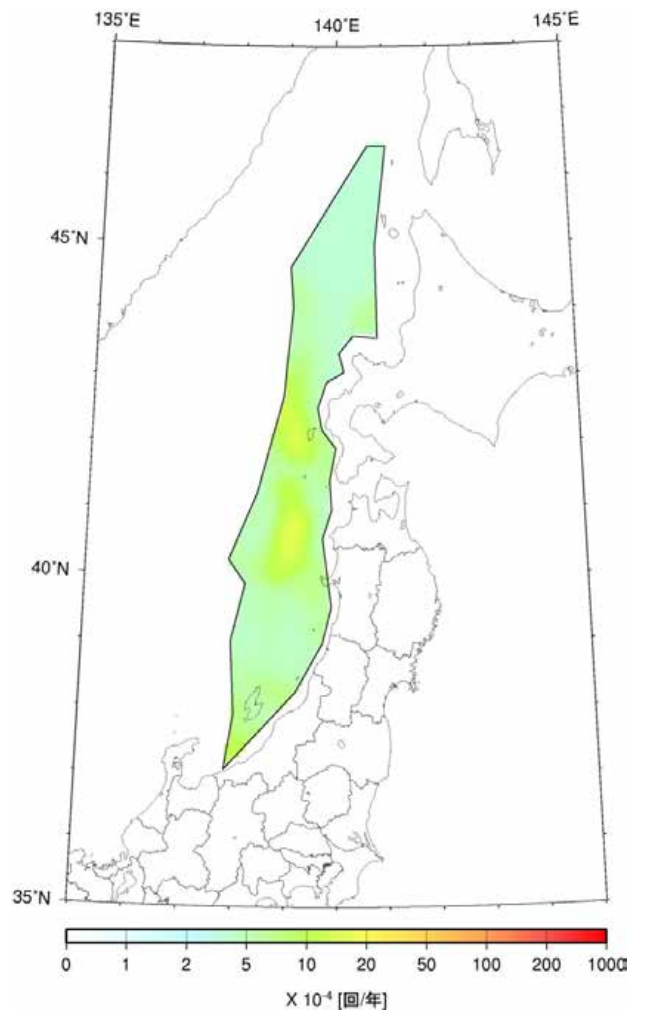
図 2. 4. 5. 6-18 日本海東縁部の震源断層を予め特定しにくい地震の発生頻度（0.1 度四方あたり， M 5.0 以上）
