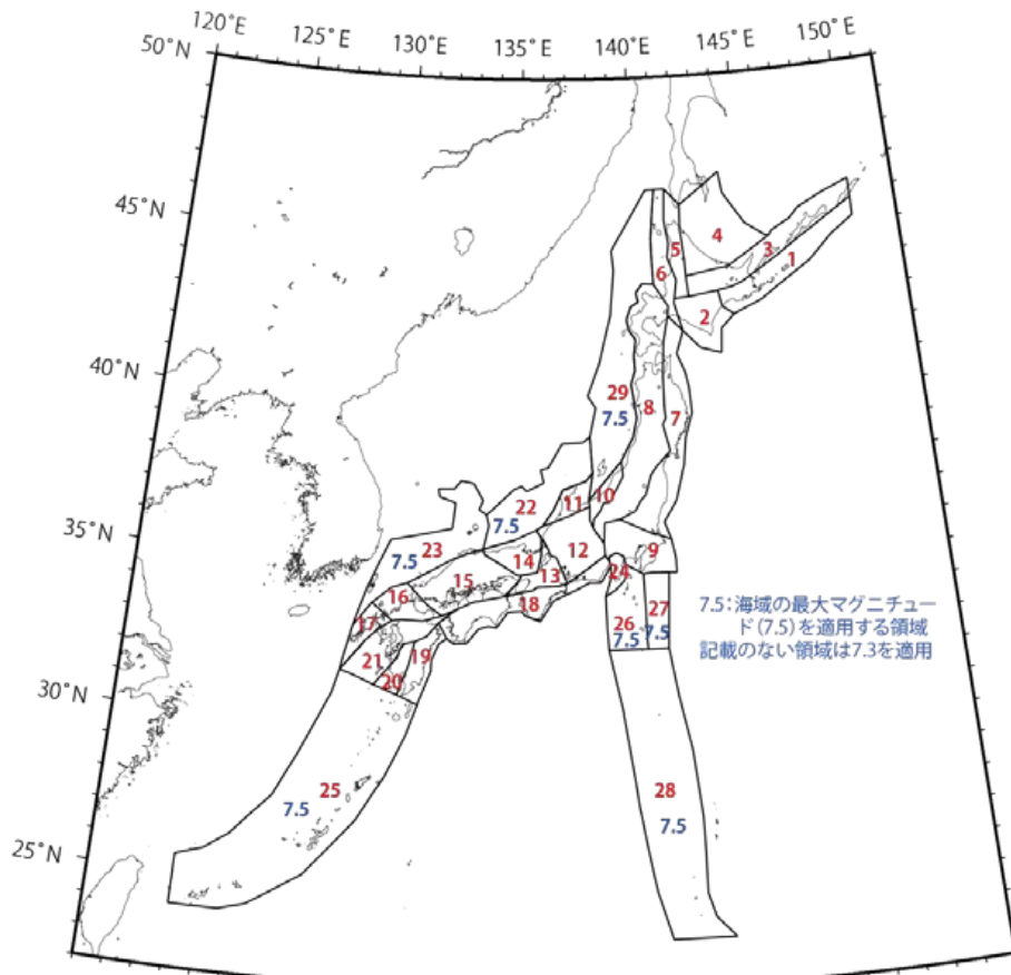
図 2.4.5.6-10 陸域の震源断層を予め特定しにくい地震の最大マグニチュード
