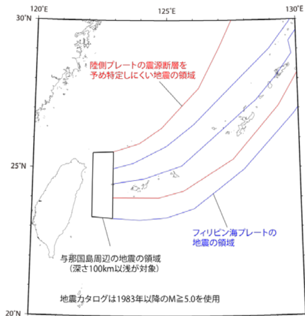
図 2.4.6.2-1 南西諸島付近の震源を特定しにくい地震の地域区分，および頻度算定に用いる地震カタログ
