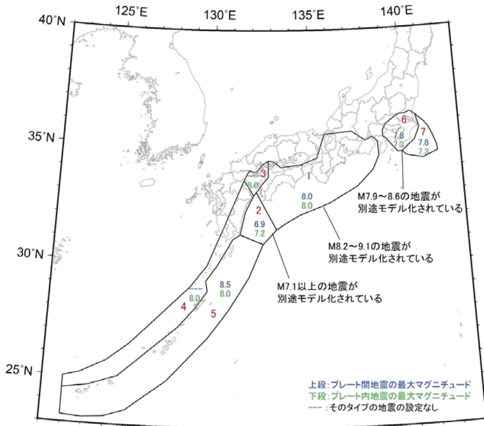
図 2. 4. 4. 3-6 フィリピン海プレートの震源断層を予め特定しにくい地震の最大マグニチュード
