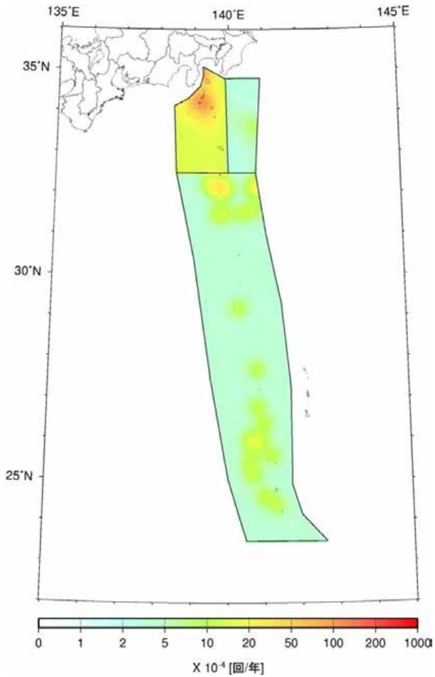
図 2.4.5.6-25 伊豆諸島以南の震源断層を予め特定しにくい地震の発生頻度 (0.1 度四方あたり, M5.0 以上)
