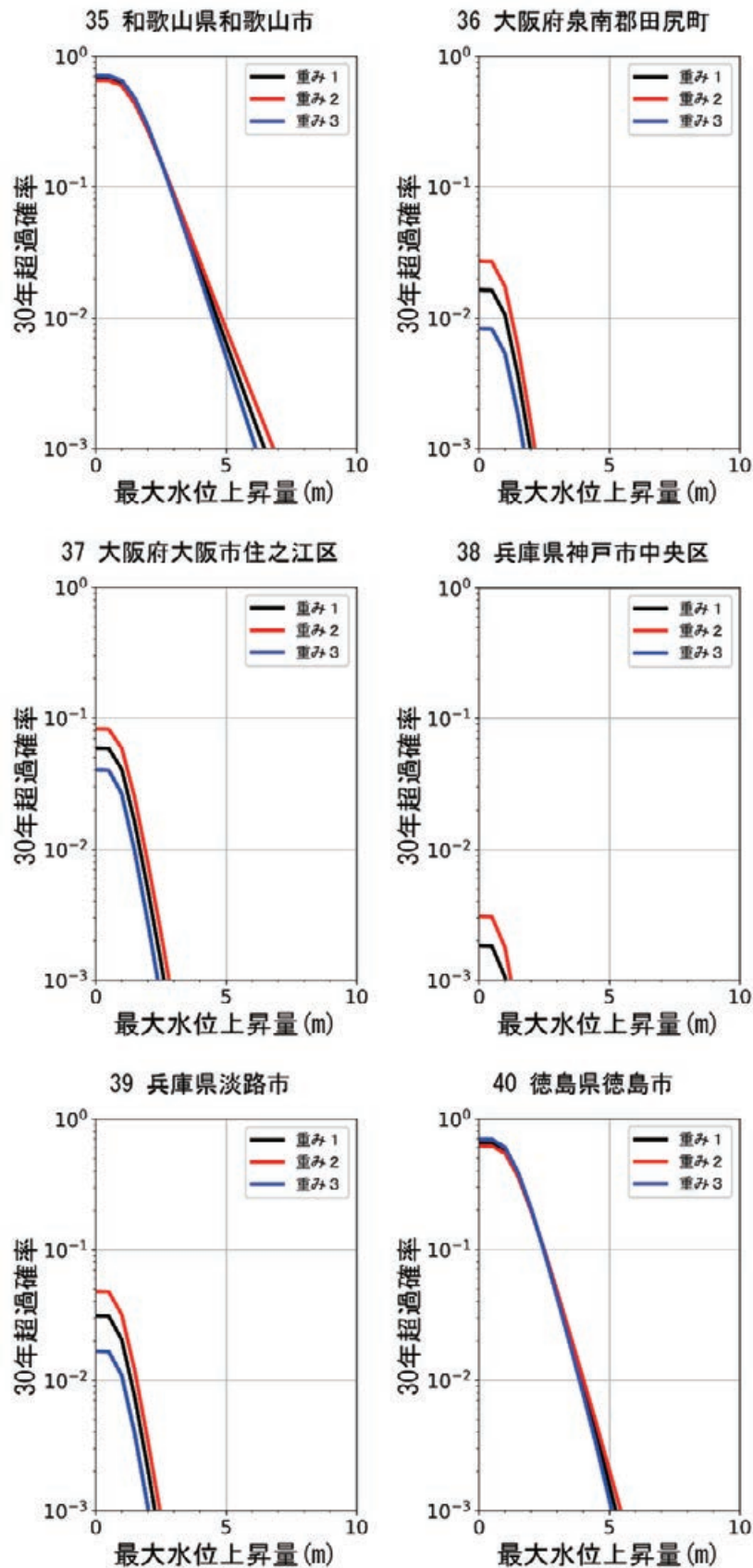
図 8.5.2-13 異なる 3 種類の重みを用いた和歌山県和歌山市，大阪府泉南郡田尻町，大阪府大阪市住之江区，兵庫県神戸市中央区，兵庫県淡路市，徳島県徳島市でのハザードカーブ比較
