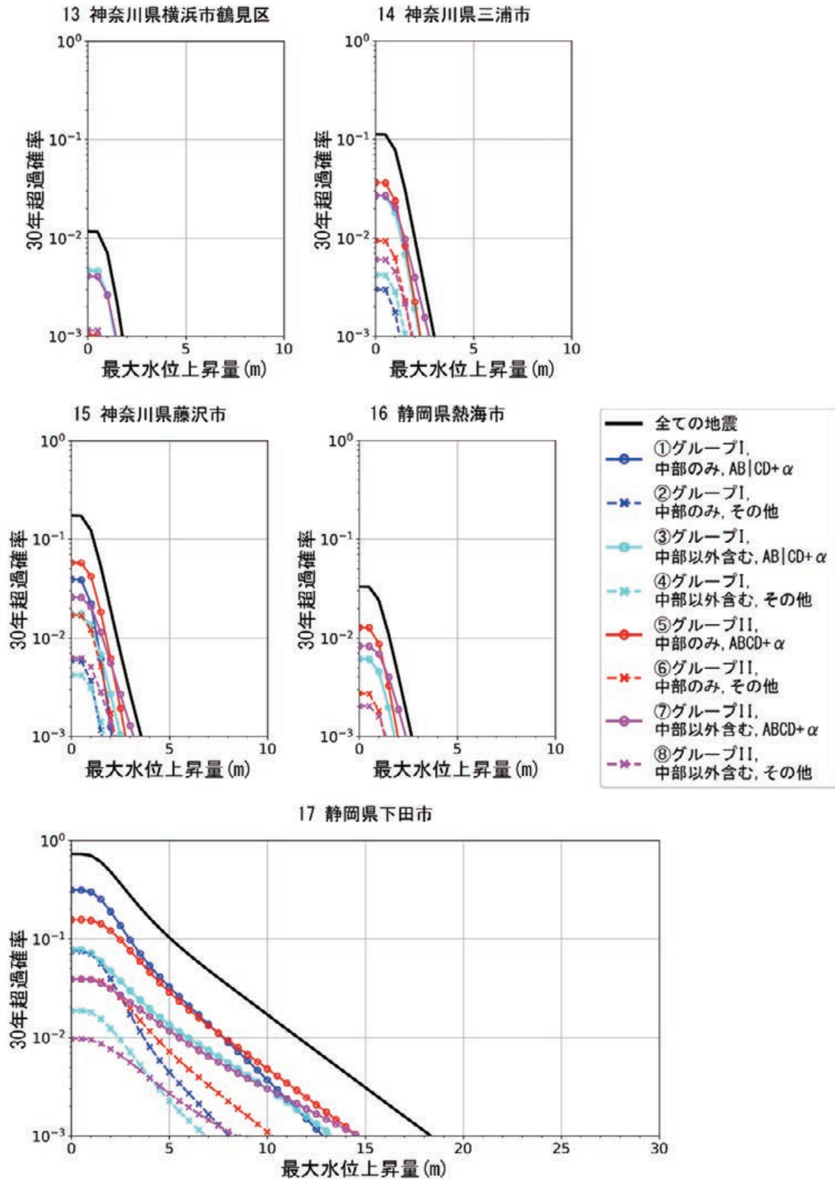
図 8.4.1-5 神奈川県横浜市鶴見区, 神奈川県三浦市, 神奈川県藤沢市, 静岡県熱海市, 静岡県下田市でのハザードカーブ
