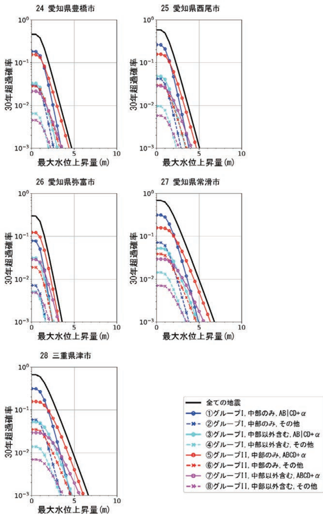
図 8.4.1-8 愛知県豊橋市, 愛知県西尾市, 愛知県弥富市, 愛知県常滑市, 三重県津市でのハザードカーブ
