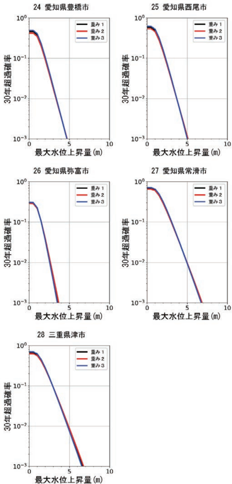
図 8.5.2-10 異なる 3 種類の重みを用いた愛知県豊橋市，愛知県西尾市，愛知県弥富市，愛知県常滑市，三重県津市でのハザードカーブ比較
