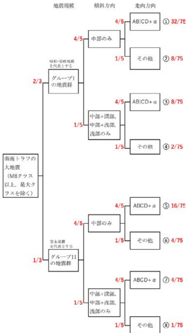
図 8.3.4-1 8つの地震カテゴリに分けられた震源域パターン。各種別の分岐点に表示された赤字は重みの配分比率。
