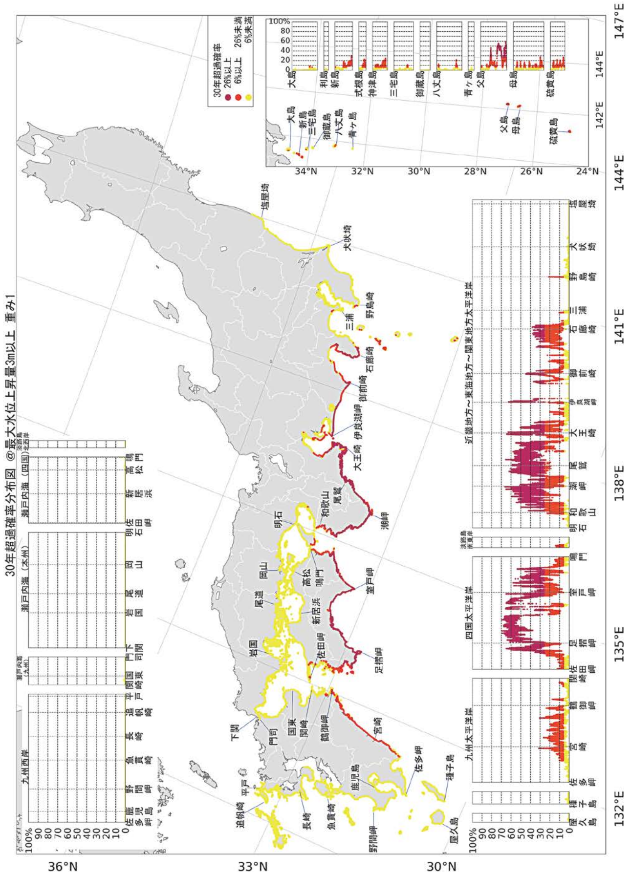
図 9.1-1 30年超過確率分布図. 最大水位上昇量3 m 以上. 地震調査委員会(2020)と同じ3区分からなるカラースケールを使用.
