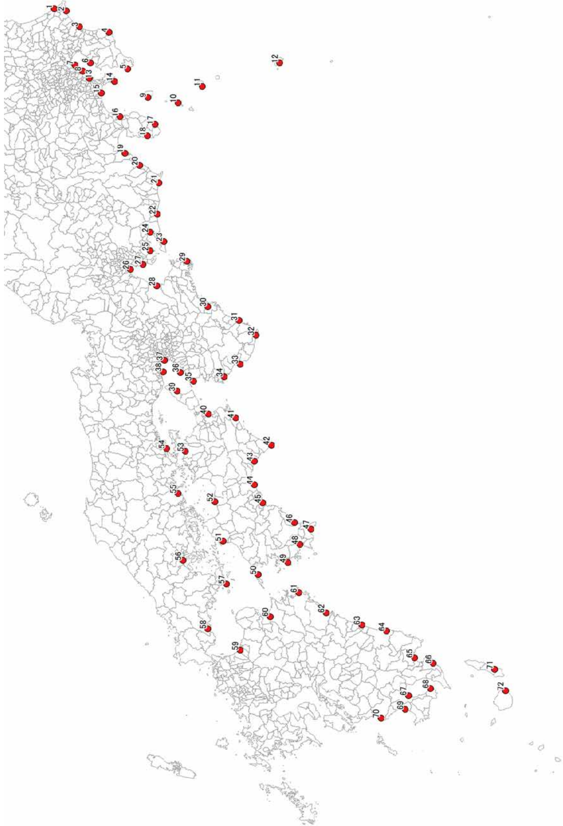
図 8.4.1-1 南海トラフ沿いに設定されたハザード評価標本点
