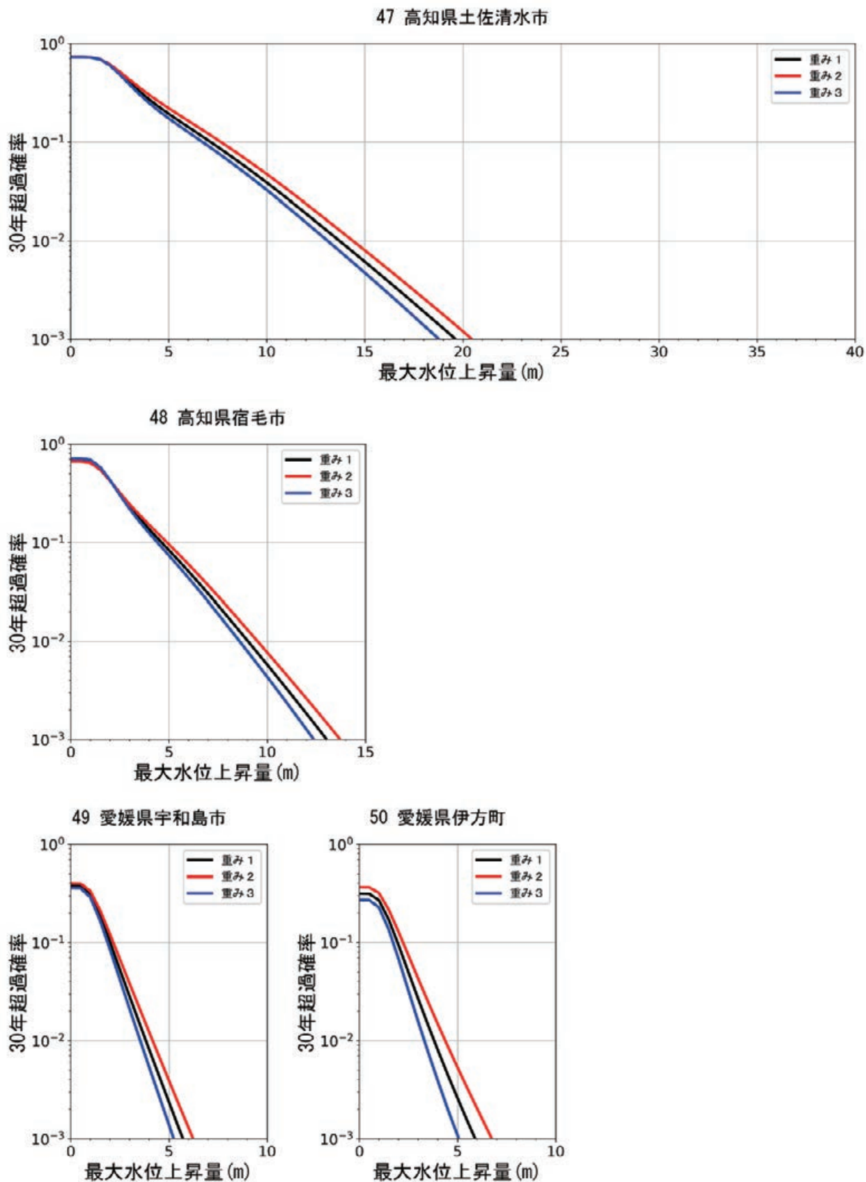
図 8.5.2-16 異なる 3 種類の重みを用いた高知県土佐清水市，高知県宿毛市，愛媛県宇和島市，愛媛県伊方町でのハザードカーブ比較
