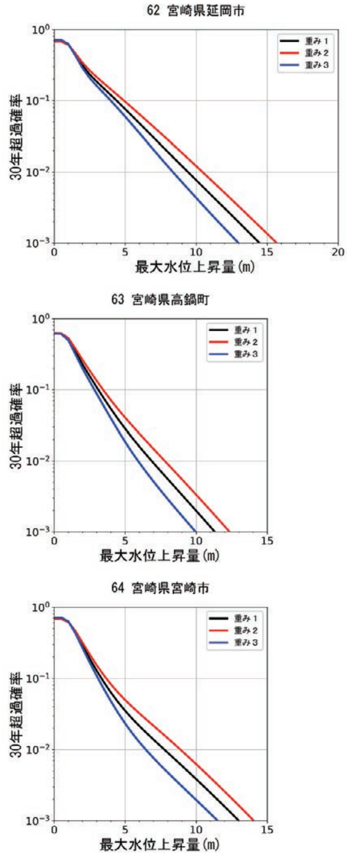
図 8.5.2-19 異なる 3 種類の重みを用いた宮崎県延岡市，宮崎県高鍋町，宮崎県宮崎市でのハザードカーブ比較
