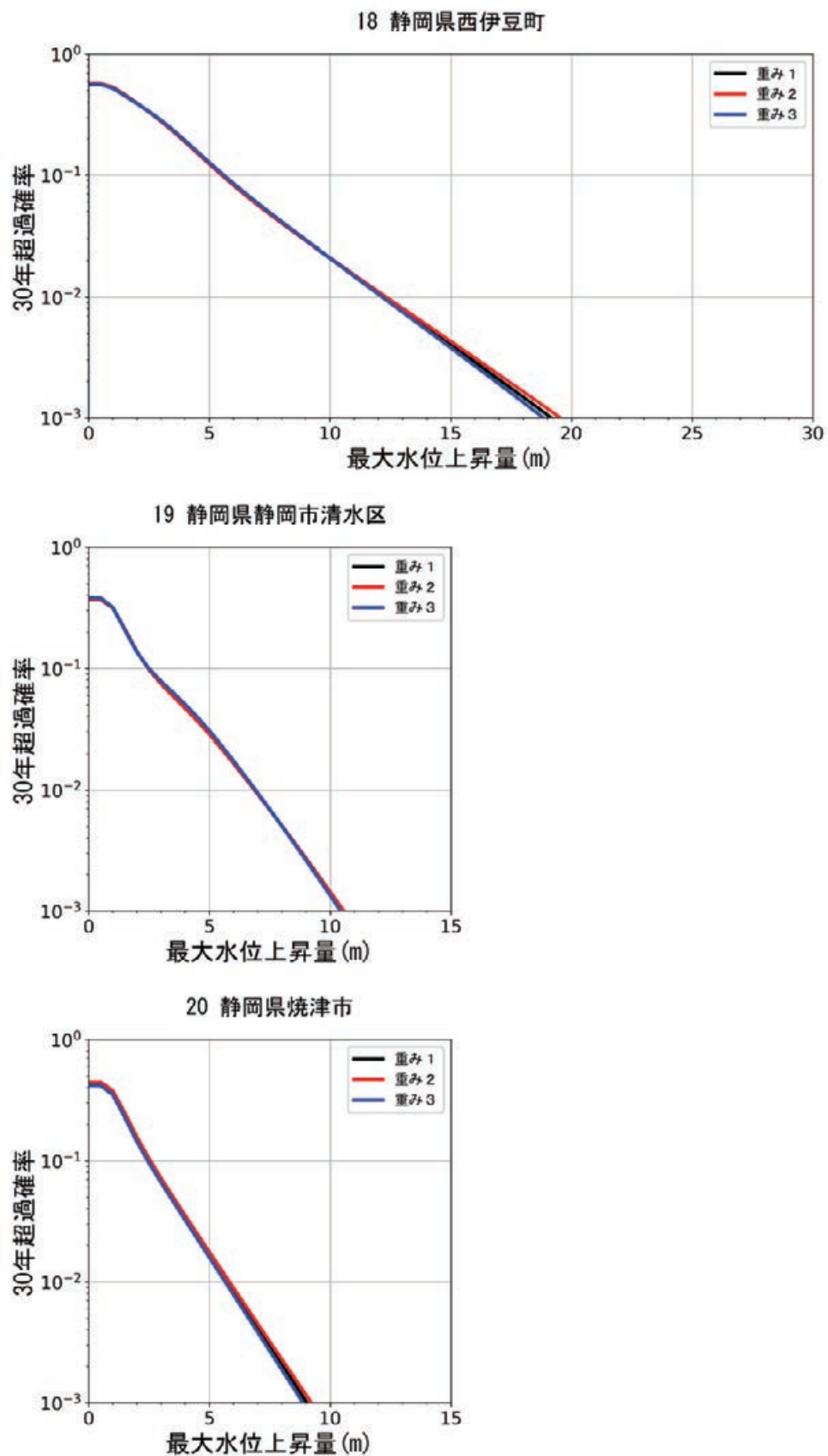
図 8.5.2-8 異なる 3 種類の重みを用いた静岡県西伊豆町，静岡県静岡市清水区，静岡県焼津市でのハザードカーブ比較
