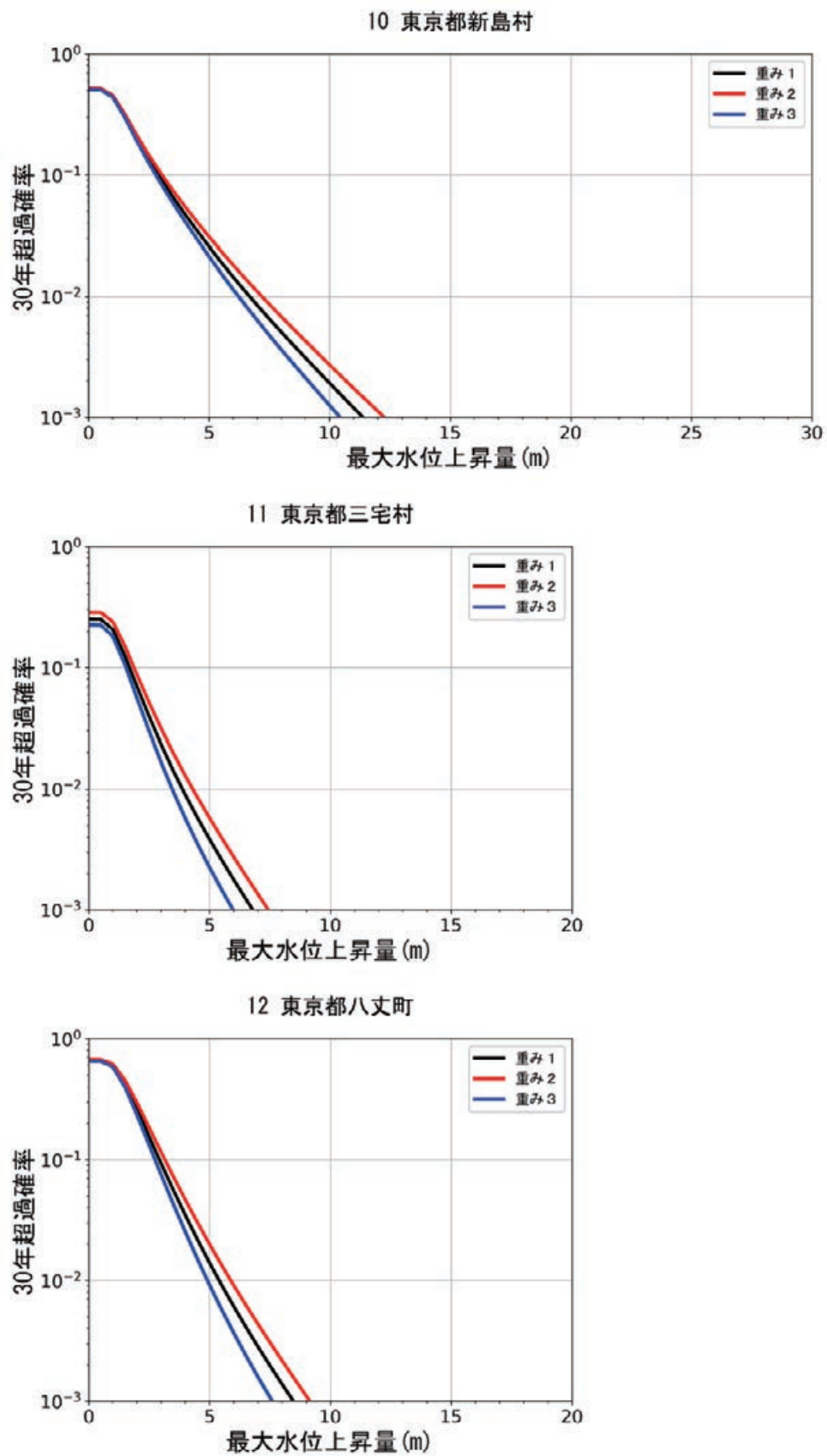
図 8.5.2-6 異なる 3 種類の重みを用いた東京都新島村，東京都三宅村，東京都八丈町でのハザードカーブ比較
