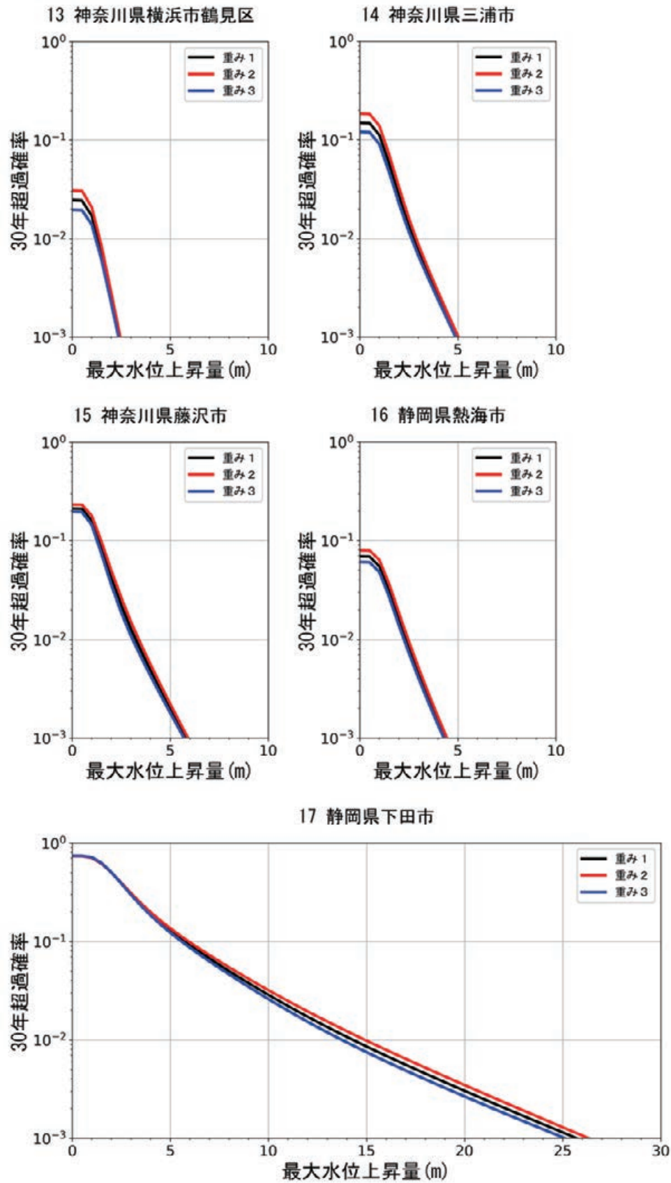
図 8.5.2-7 異なる 3 種類の重みを用いた神奈川県横浜市鶴見区，神奈川県三浦市，神奈川県藤沢市，静岡県熱海市，静岡県下田市でのハザードカーブ比較
