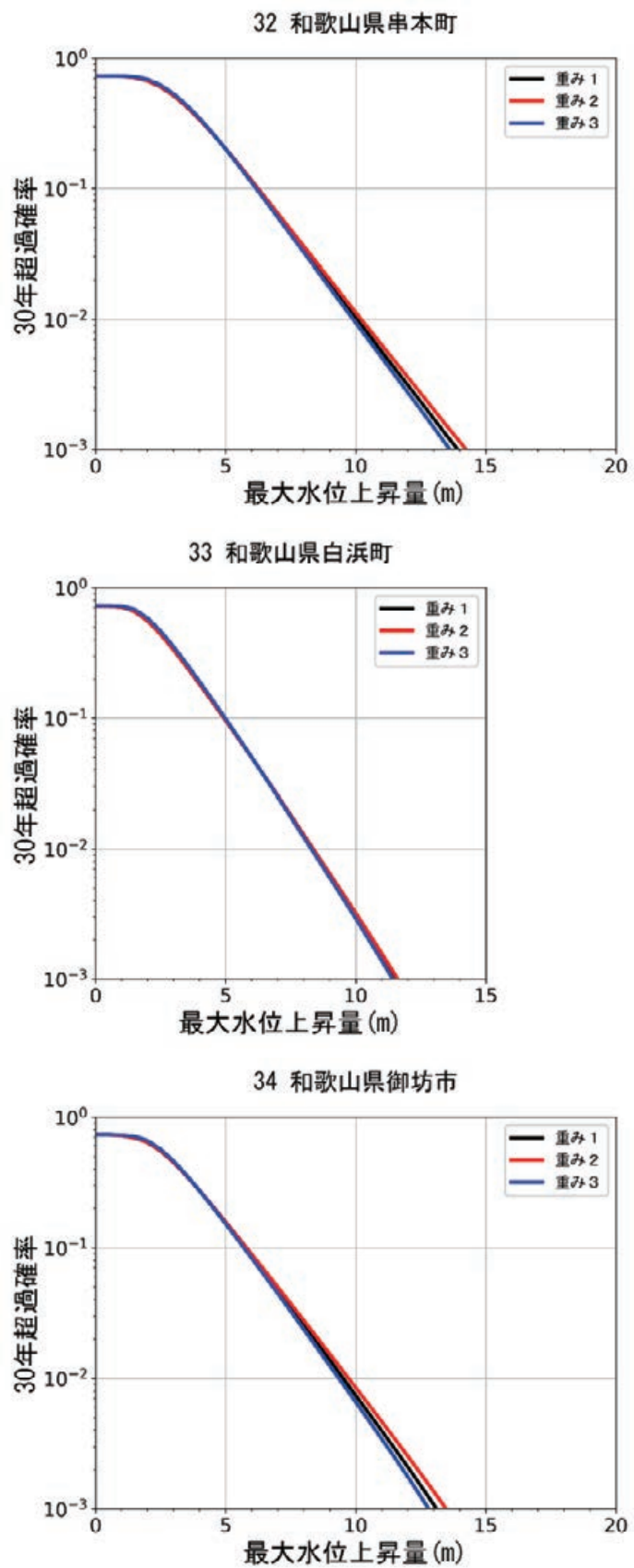
図 8.5.2-12 異なる 3 種類の重みを用いた和歌山県串本町，和歌山県白浜町，和歌山県御坊市でのハザードカーブ比較
