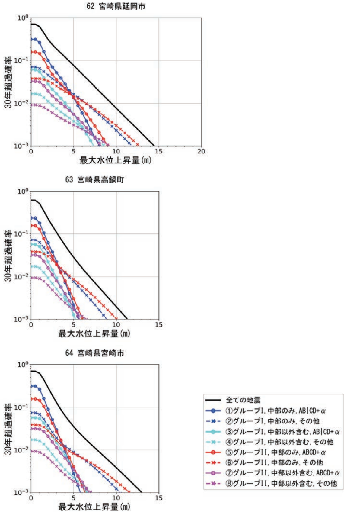
図 8.4.1-17 宮崎県延岡市, 宮崎県高鍋町, 宮崎県宮崎市でのハザードカーブ
