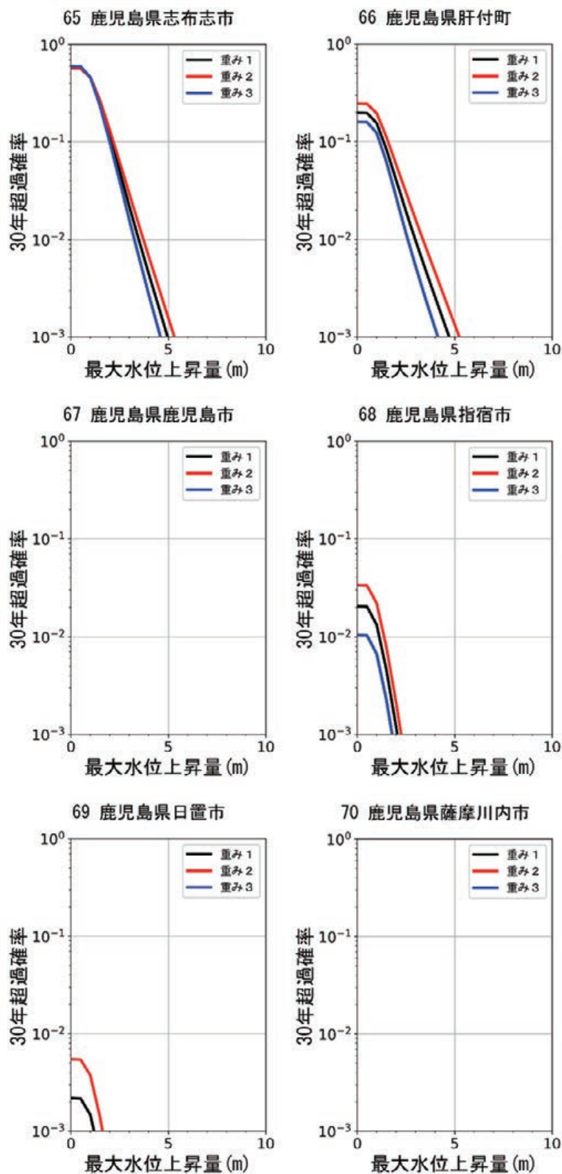
図 8.5.2-20 異なる 3 種類の重みを用いた鹿児島県志布志市，鹿児島県肝付町，鹿児島県鹿児島市，鹿児島県指宿市，鹿児島県日置市，鹿児島県薩摩川内市でのハザードカーブ比較
