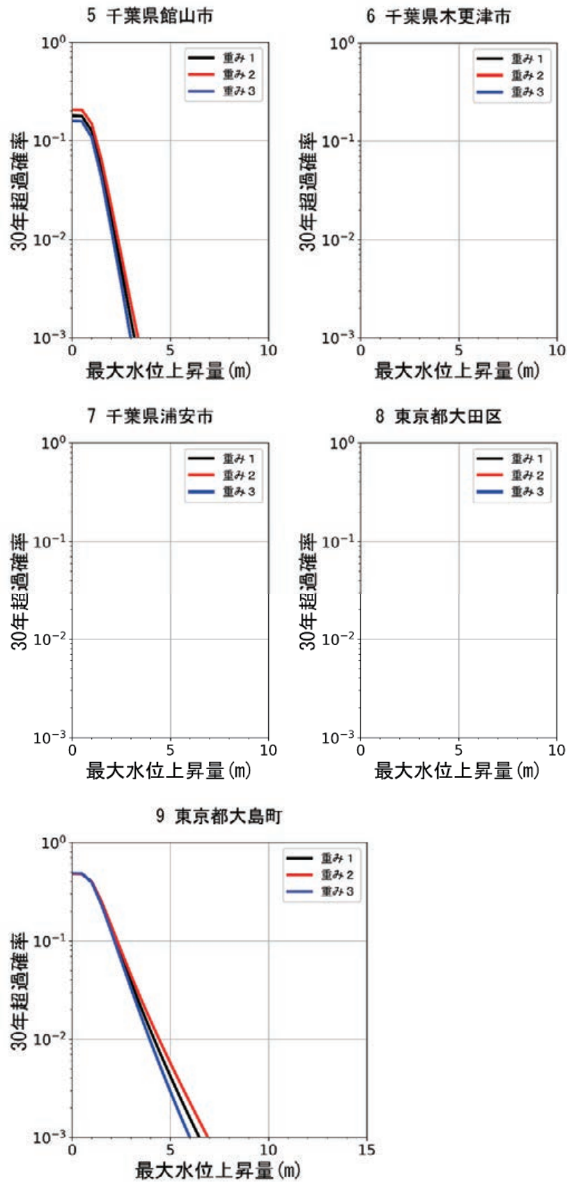
図 8.5.2-5 異なる 3 種類の重みを用いた千葉県館山市，千葉県木更津市，千葉県浦安市，東京都大田区，東京都大島町でのハザードカーブ比較
