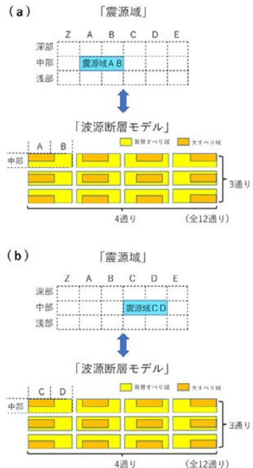
図 8.1.1-1 震源域と波源断層モデルの対応関係。 この例では、上段の (a) の震源域 AB に、12 通りの波源断層モデルが対応し、下段の (b) の震源域 CD にも、12 通りの波源断層モデルが対応している。
