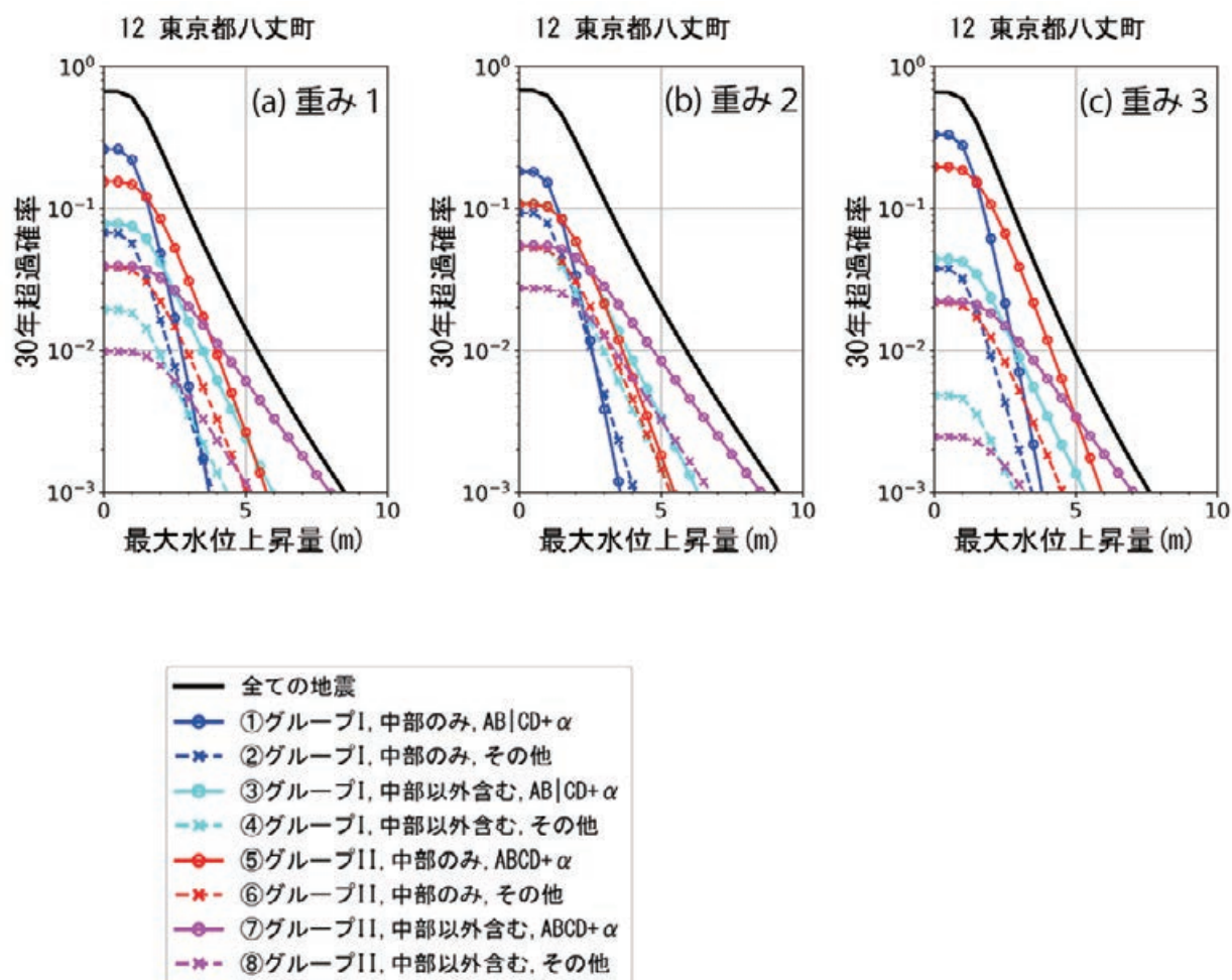
図 8.5.2-22 東京都八丈町 (No.12) のハザードカーブとその再分解表現. (a) 重み 1 を適用した場合. (b) 重み 2 を適用した場合. (c) 重み 3 を適用した場合.
