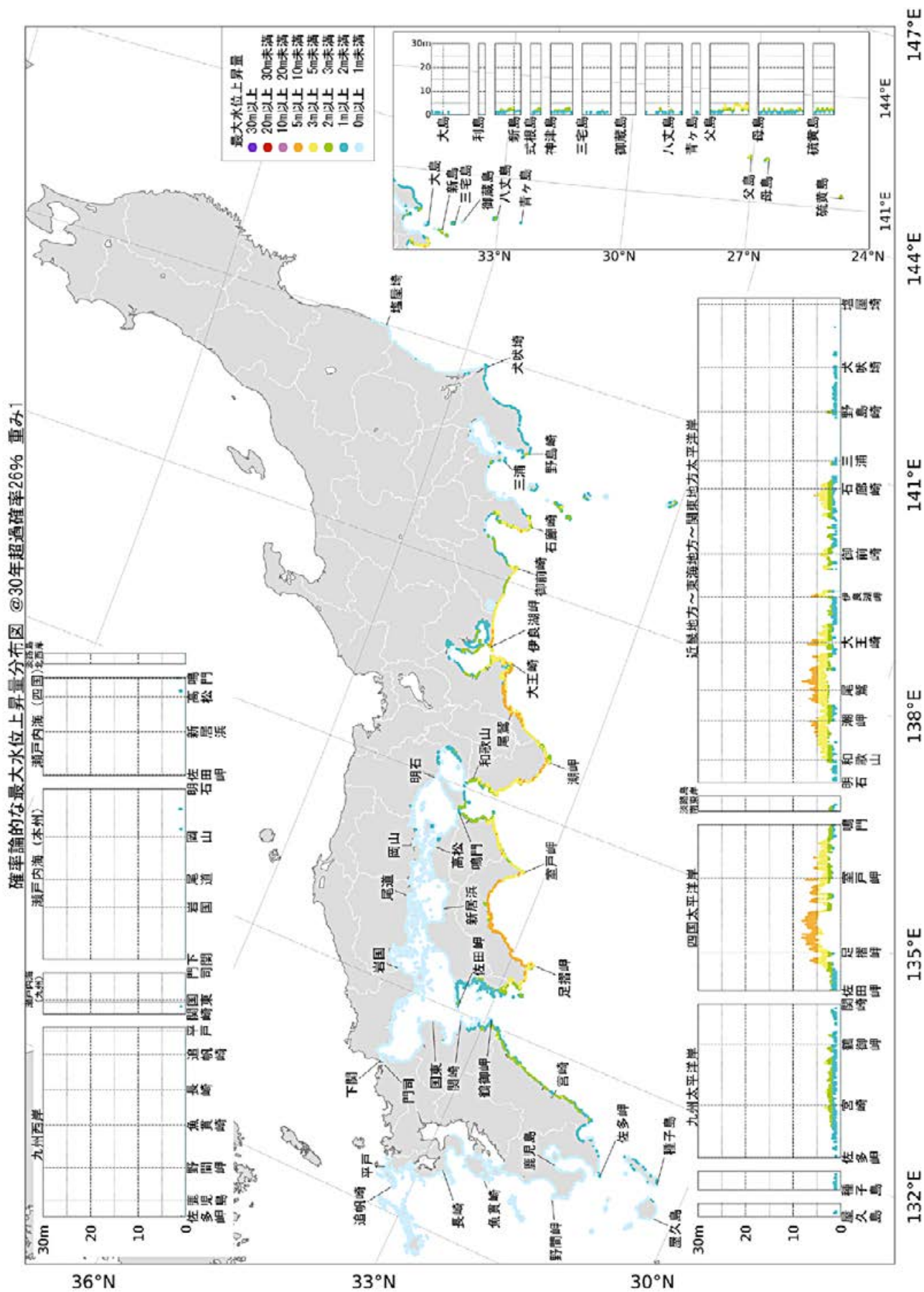
図 9.2-1 確率論的な最大水位上昇量分布図. 30 年超過確率 26%.
