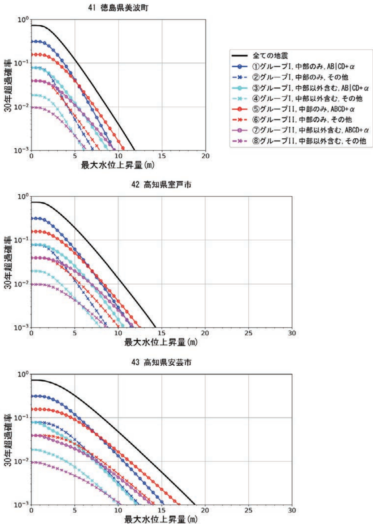
図 8.4.1-12 徳島県美波町, 高知県室戸市, 高知県安芸市でのハザードカーブ
