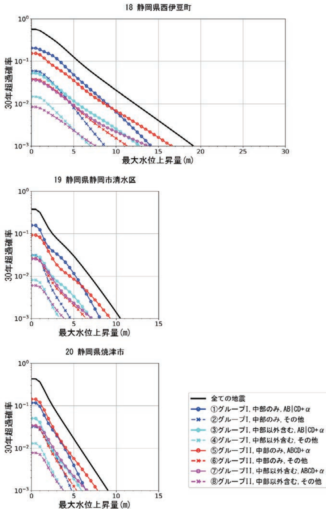
図 8.4.1-6 静岡県西伊豆町，静岡県静岡市清水区，静岡県焼津市でのハザードカーブ
