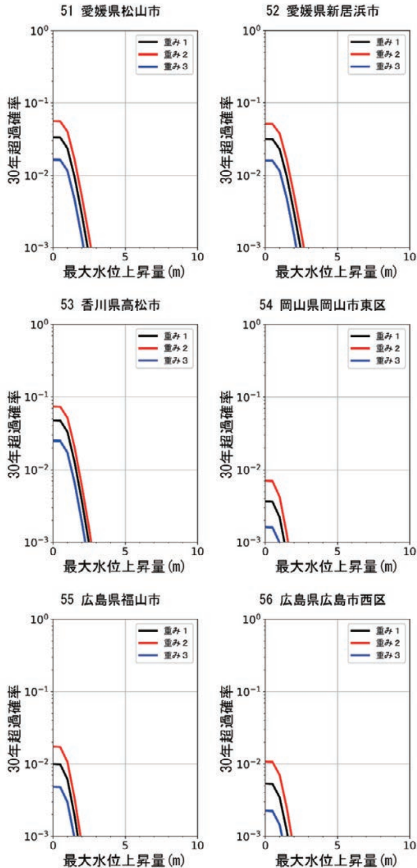
図 8.5.2-17 異なる 3 種類の重みを用いた愛媛県松山市、愛媛県新居浜市、香川県高松市、岡山県岡山市東区、広島県福山市、広島県広島市西区でのハザードカーブ比較
