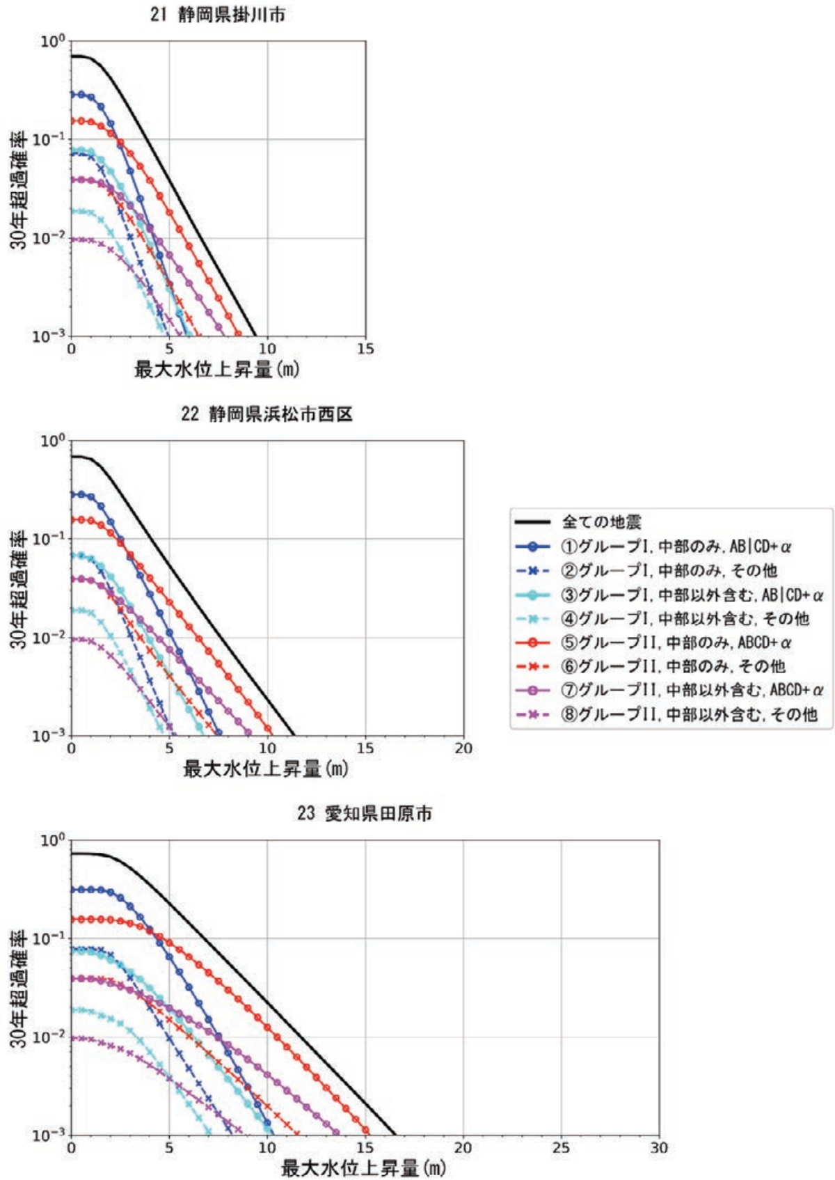
図 8.4.1-7 静岡県掛川市，静岡県浜松市西区，愛知県田原市でのハザードカーブ
