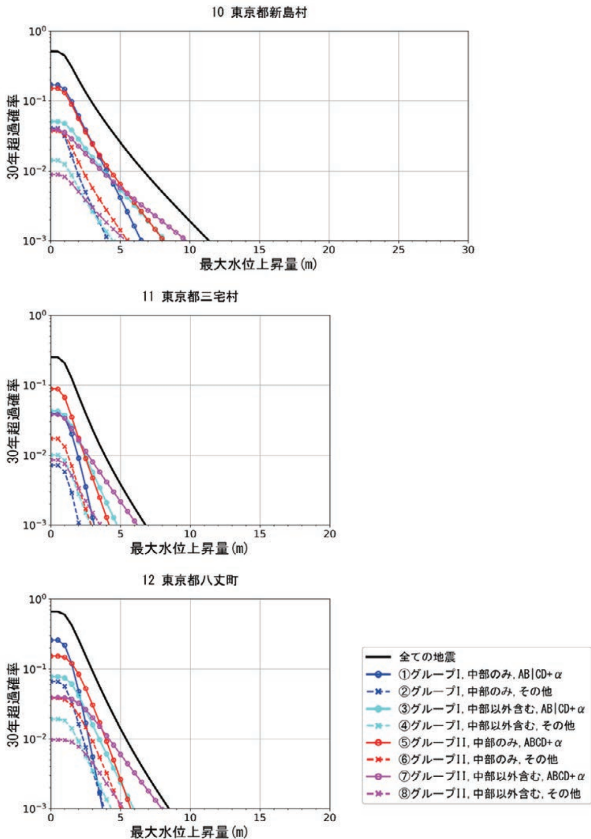
図 8.4.1-4 東京都新島村，東京都三宅村，東京都八丈町でのハザードカーブ
