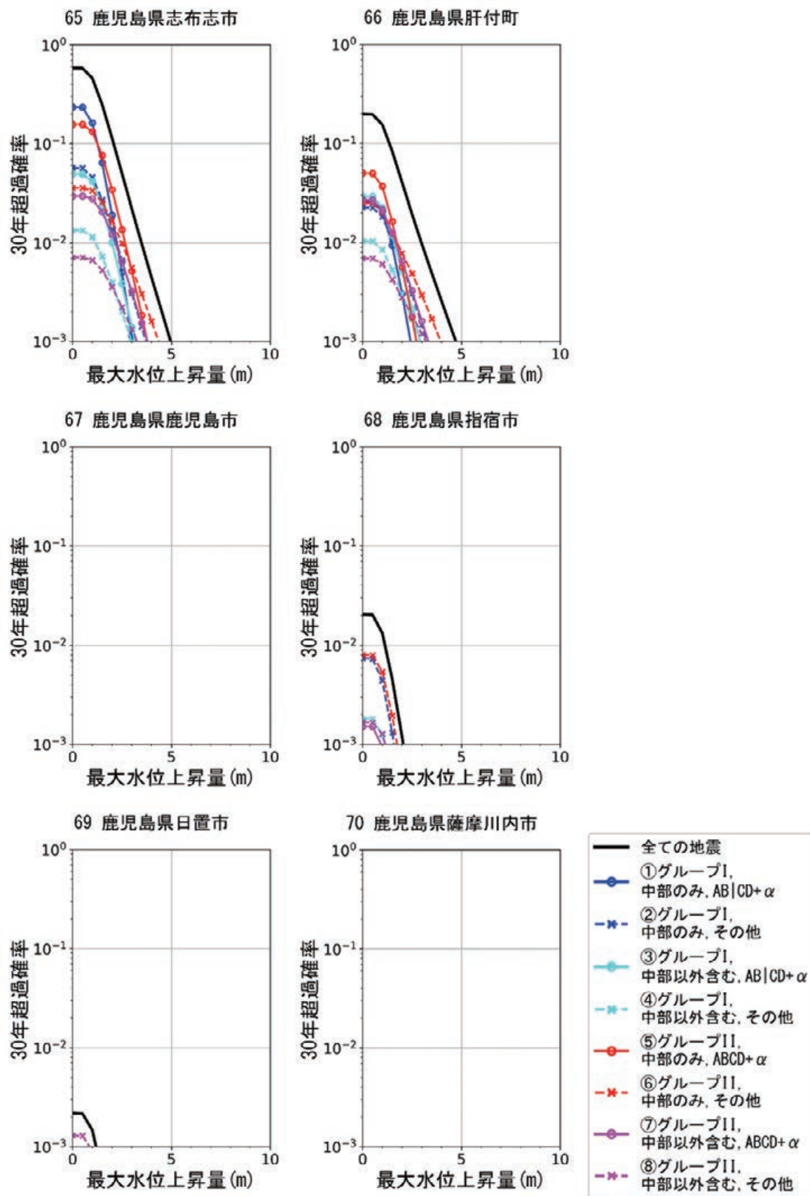
図 8.4.1-18 鹿児島県志布志市，鹿児島県肝付町，鹿児島県鹿児島市，鹿児島県指宿市，鹿児島県日置市，鹿児島県薩摩川内市のハザードカーブ
