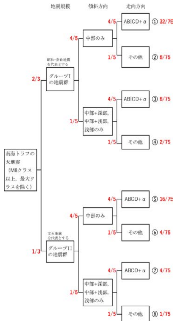
図 8.5.2-1 「重み 1」を適用した 9 つの地震カテゴリーへの重みの配分枝図(図 8.3.4-1 再掲)
