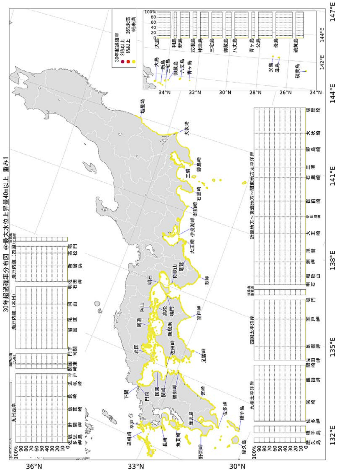
図 9.1-5 30 年超過確率分布図. 最大水位上昇量 40 m 以上. 地震調査委員会 (2020) と同じ 3 区分からなるカースケールを使用.
