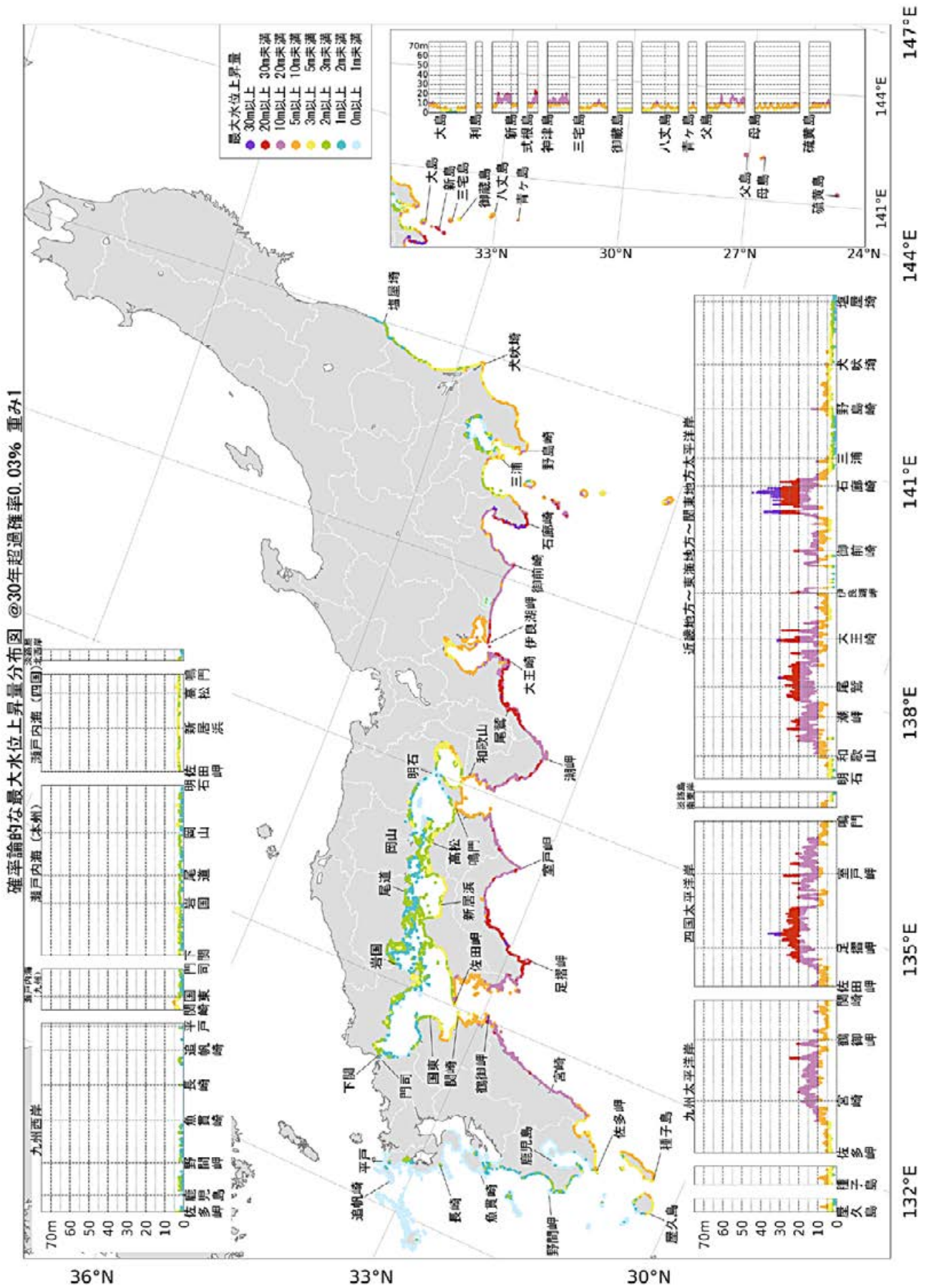
図 9.2-5 確率論的な最大水位上昇量分布図. 30 年超過確率 0.03%.
