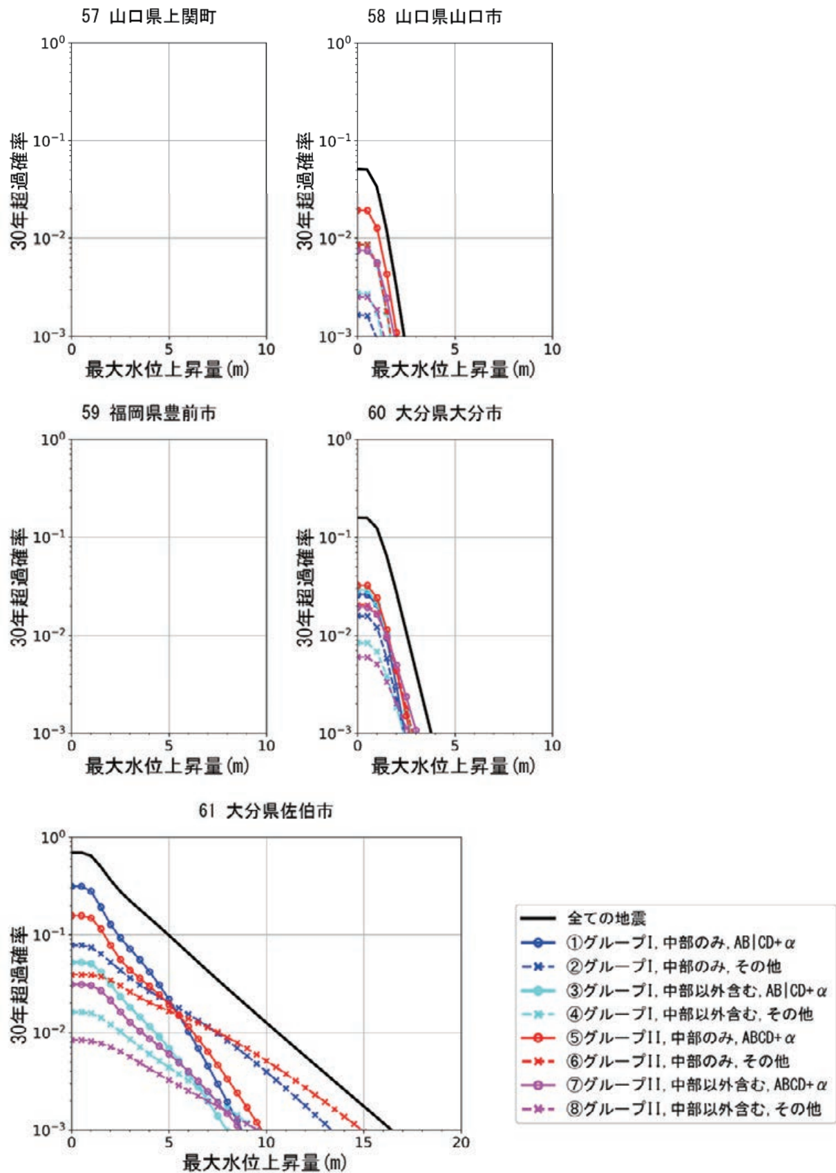
図 8.4.1-16 山口県上関町, 山口県山口市, 福岡県豊前市, 大分県大分市, 大分県佐伯市でのハザードカーブ
