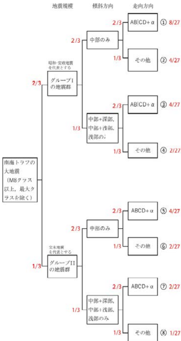
図 8.5.2-2 「重み 2」を適用した 9 つの地震カテゴリへの重みの配分枝図). 「重み 1」を適用した枝図 (図 8.5.2-1) と比べて, 「傾斜方向」および「走向方向」の枝で, 重み配分が異なっている.
