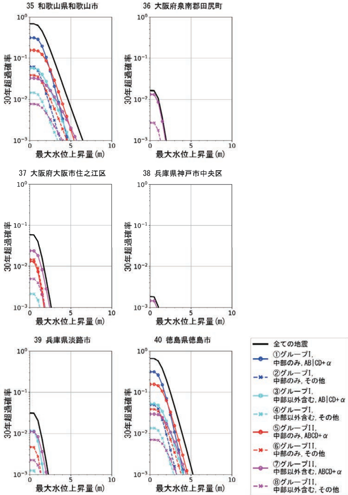
図 8.4.1-11 和歌山県和歌山市, 大阪府泉南郡田尻町, 大阪府大阪市住之江区, 兵庫県神戸市中央区, 兵庫県淡路市, 徳島県徳島市でのハザードカーブ
