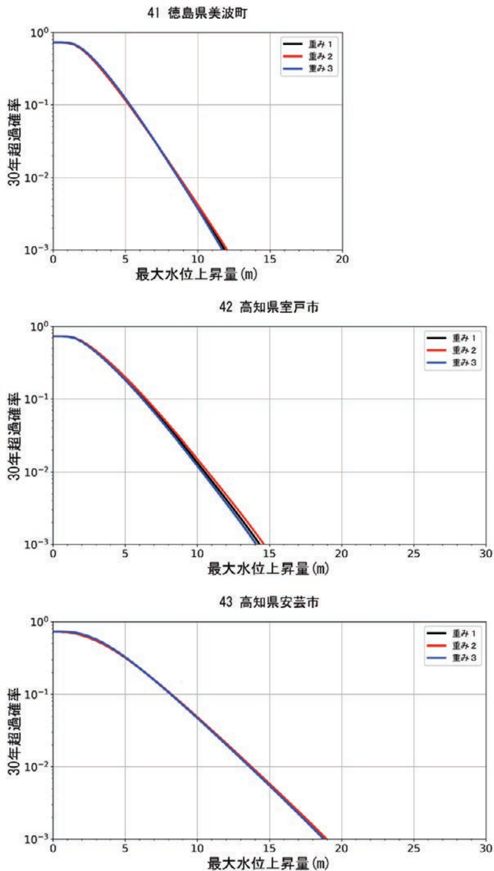
図 8.5.2-14 異なる 3 種類の重みを用いた徳島県美波町，高知県室戸市，高知県安芸市でのハザードカーブ比較
