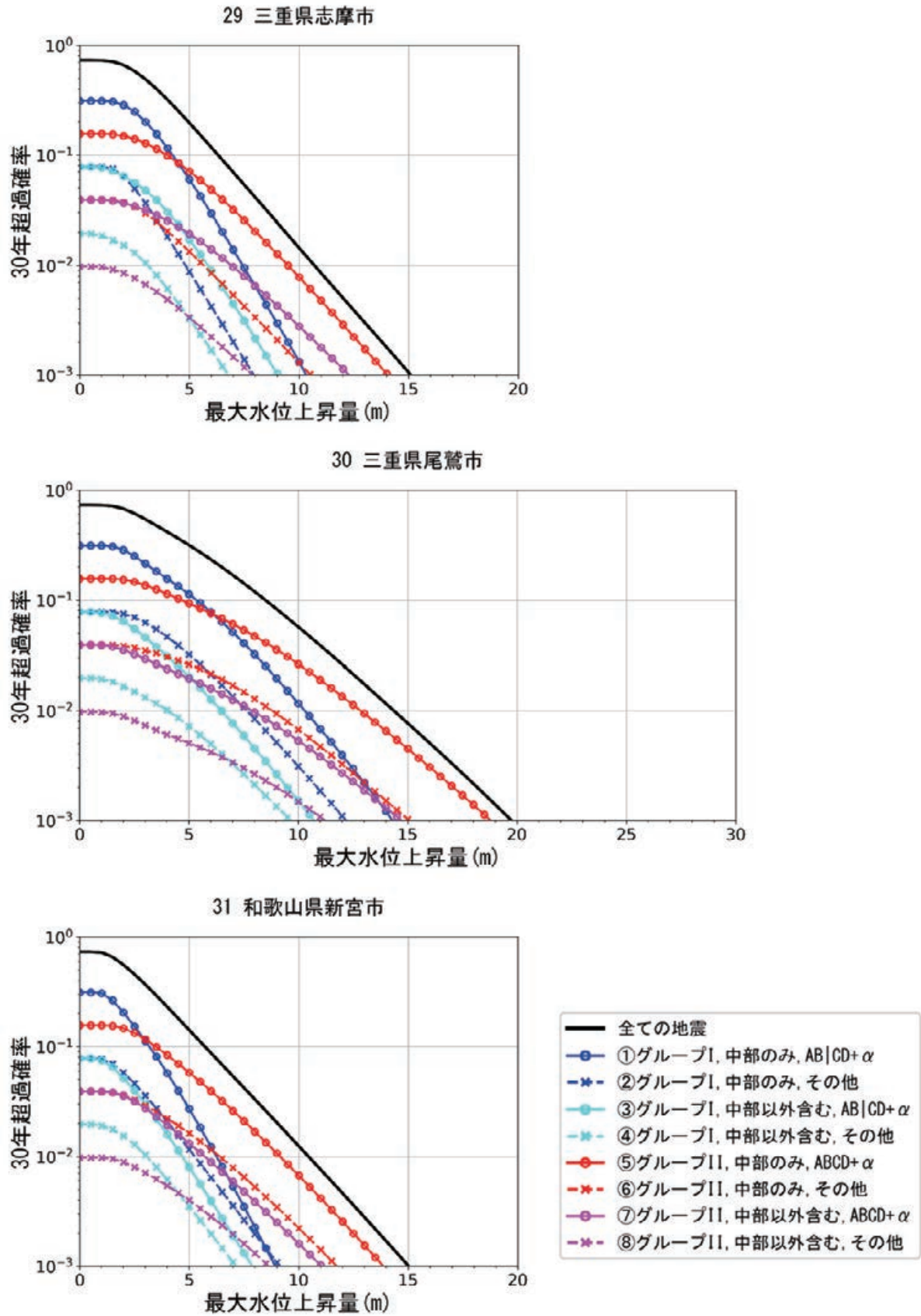
図 8.4.1-9 三重県志摩市, 三重県尾鷲市, 和歌山県新宮市でのハザードカーブ
