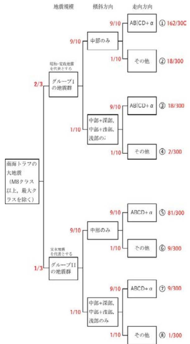
図 8.5.2-3 「重み 3」を適用した 9 つの地震カテゴリへの重みの配分枝図). 「重み 1」を適用した枝図 (図 8.5.2-1) および「重み 2」を適用した枝図 (図 8.5.2-2) と比べて, 「傾斜方向」および「走向方向」の枝で, 重み配分が異なっている.
