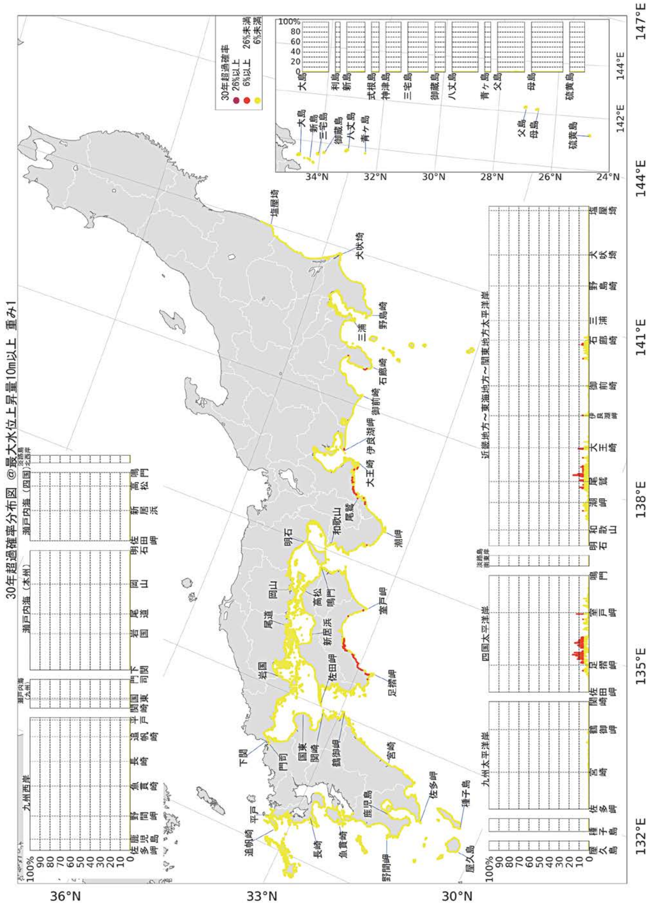
図 9.1-3 30年超過確率分布図. 最大水位上昇量 10 m 以上. 地震調査委員会(2020)と同じ3区分からなるカースケールを使用.
