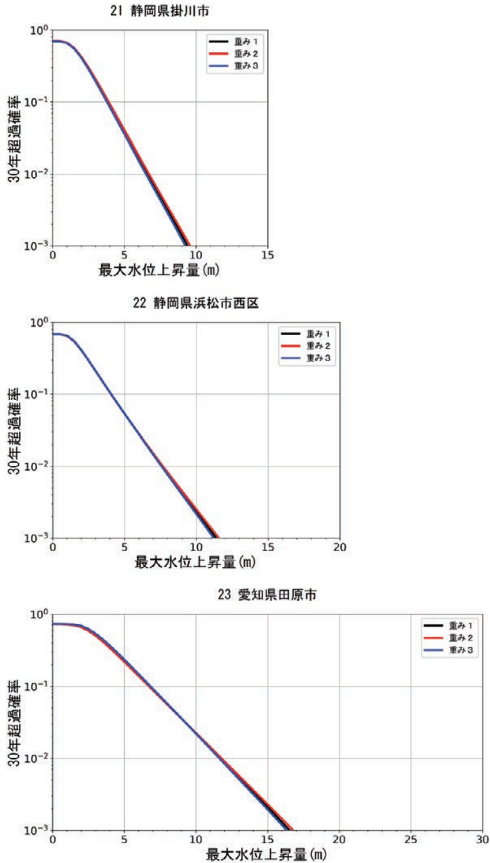
図 8.5.2-9 異なる 3 種類の重みを用いた静岡県掛川市，静岡県浜松市西区，愛知県田原市でのハザードカーブ比較
