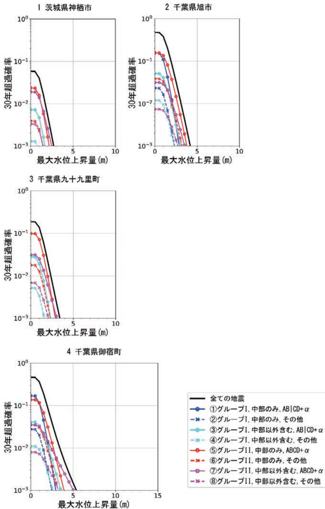
図 8.4.1-2 茨城県神栖市, 千葉県旭市, 千葉県九十九里町, 千葉県御宿町でのハザードカーブ
