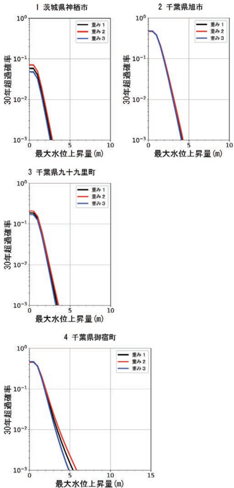
図 8.5.2-4 異なる 3 種類の重みを用いた茨城県神栖市，千葉県旭市，千葉県九十九里町，千葉県御宿町でのハザードカーブ比較
