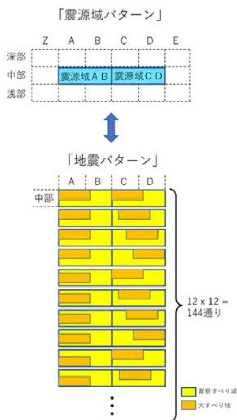
図 8.1.1-2 震源域パターンと地震パターンの対応関係。震源域 AB を持つ波源断層モデルが 12 通り、震源域 CD を持つ波源断層モデルも 12 通りの場合、震源域 AB と震源域 CD から構成される震源域パターンに対応する地震パターンは 12 \times 12 = 144 通り存在する。
