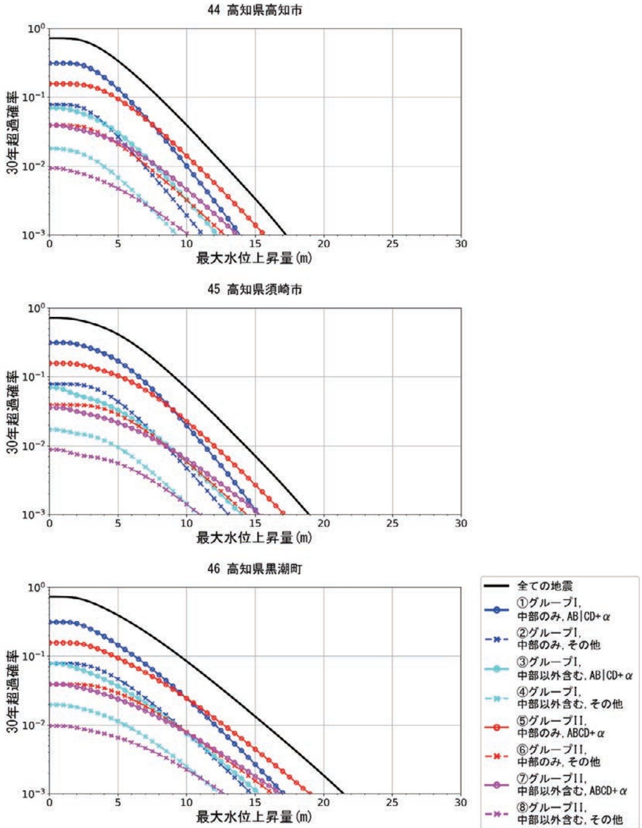
図 8.4.1-13 高知県高知市, 高知県須崎市, 高知県黒潮町でのハザードカーブ
