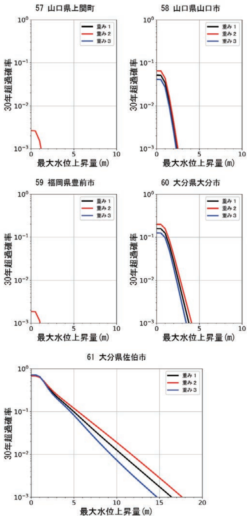
図 8.5.2-18 異なる 3 種類の重みを用いた山口県上関町，山口県山口市，福岡県豊前市，大分県大分市，大分県佐伯市でのハザードカーブ比較
