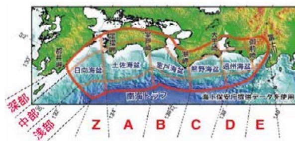
図 8.2.1-1 南海トラフ沿いで発生するプレート間地震の地震発生帯の領域区分(地震調査委員会(2013)に加筆)。
