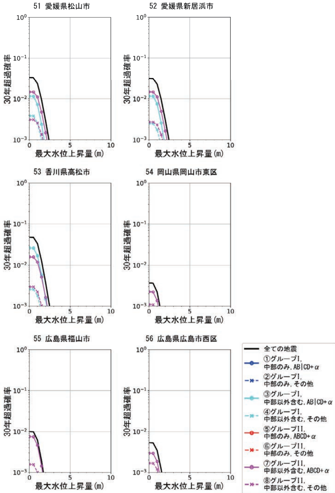
図 8.4.1-15 愛媛県松山市, 愛媛県新居浜市, 香川県高松市, 岡山県岡山市東区, 広島県福山市, 広島県広島市西区のハザードカーブ
