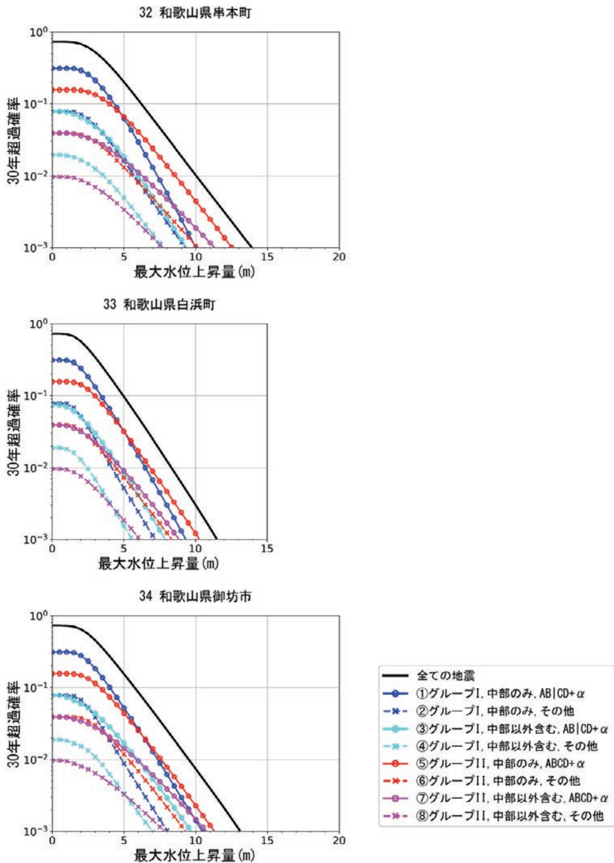
図 8.4.1-10 和歌山県串本町，和歌山県白浜町，和歌山県御坊市でのハザードカーブ
