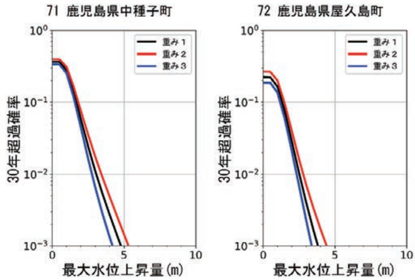
図 8.5.2-21 異なる 3 種類の重みを用いた鹿児島県中種子町，鹿児島県屋久島町でのハザードカーブ比較
