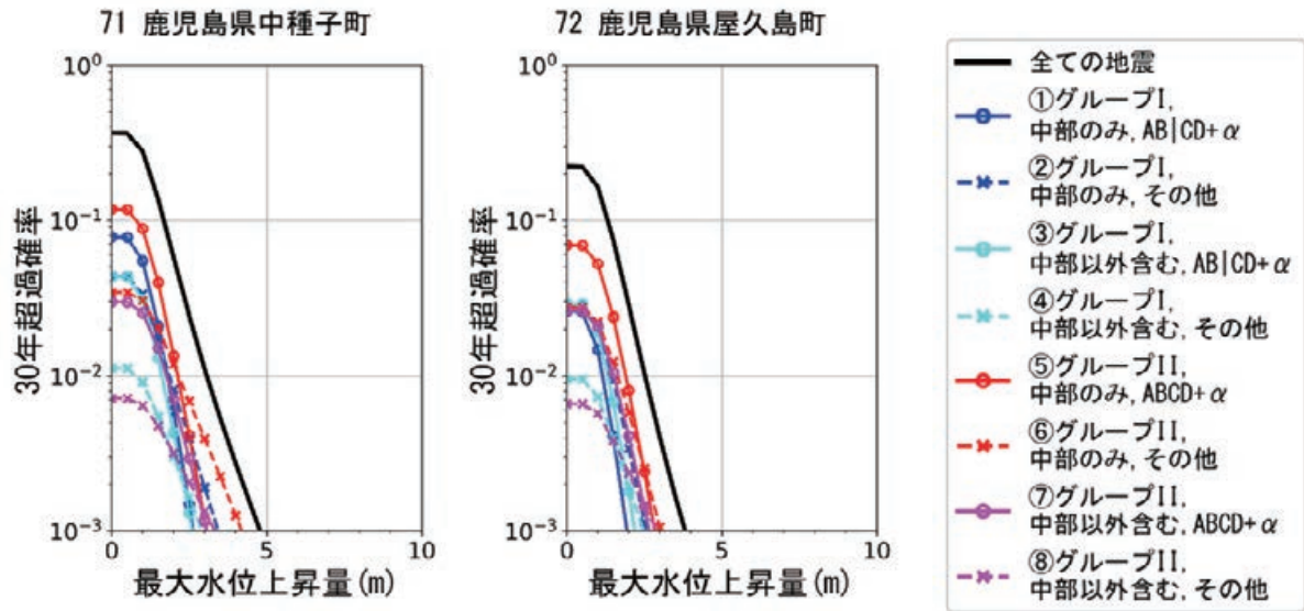
図 8.4.1-19 鹿児島県中種子町, 鹿児島県屋久島町でのハザードカーブ
