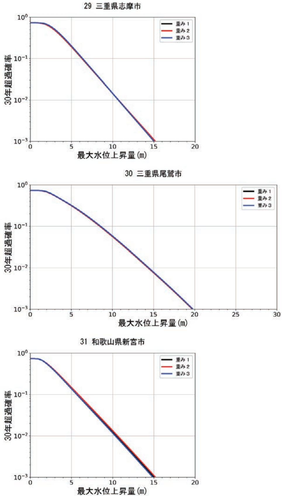
図 8.5.2-11 異なる 3 種類の重みを用いた三重県志摩市，三重県尾鷲市，和歌山県新宮市でのハザードカーブ比較
