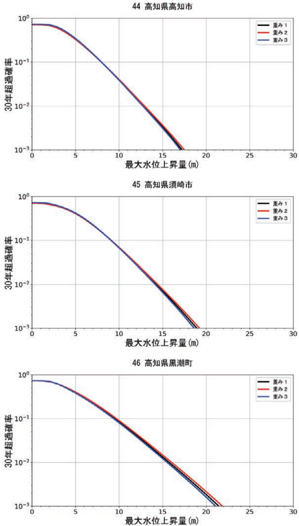
図 8.5.2-15 異なる 3 種類の重みを用いた高知県高知市，高知県須崎市，高知県黒潮町でのハザードカーブ比較
