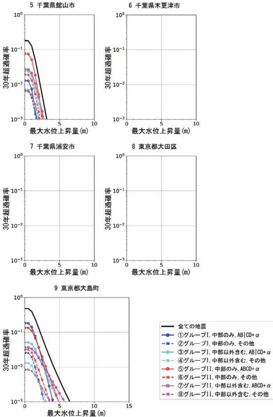
図 8.4.1-3 千葉県館山市, 千葉県木更津市, 千葉県浦安市, 東京都大田区, 東京都大島町でのハザードカーブ
