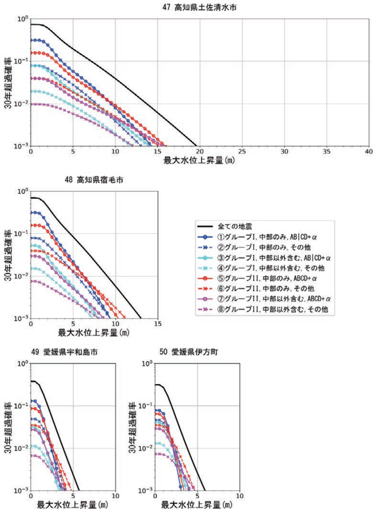
図 8.4.1-14 高知県土佐清水市，高知県宿毛市，愛媛県宇和島市，愛媛県伊方町でのハザードカーブ
