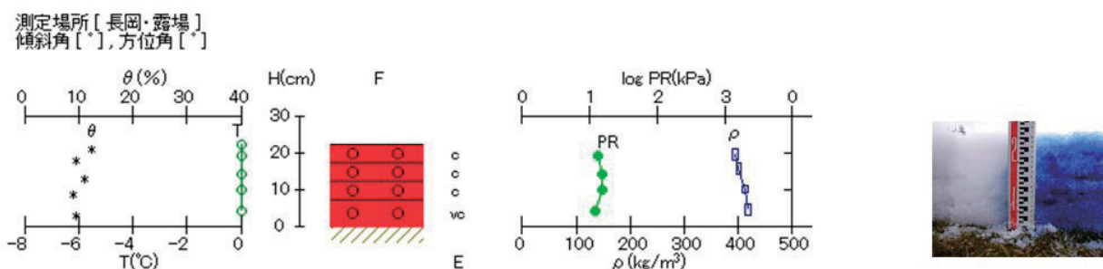
図 6.9 積雪断面観測値(長岡, 平成 31 年 2 月 21 日)
