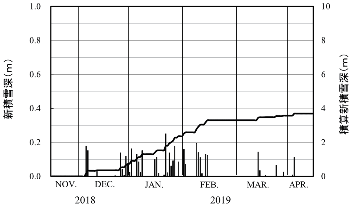
図 4.2 雪氷防災研究センターにおける新積雪深ならびに積算新積雪深の時間変化(2018/19) Fig. 4.2 Time series of the depth of newly fallen snow and its cumulative value at the SIRC (2018/19).
