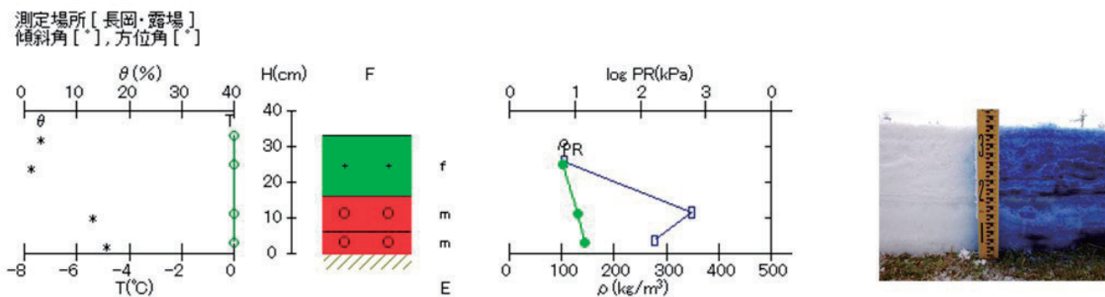
図 6.1 積雪断面観測値(長岡, 平成 31 年 1 月 3 日)
