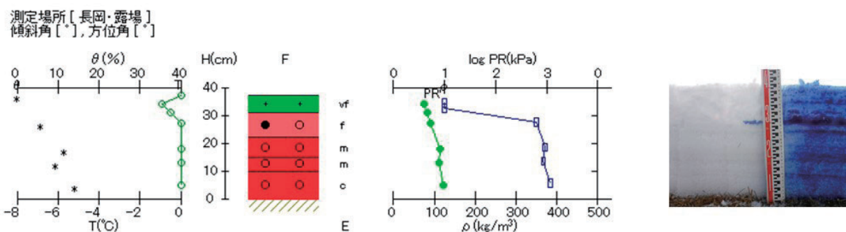
図 6.2 積雪断面観測値(長岡, 平成 31 年 1 月 10 日)
