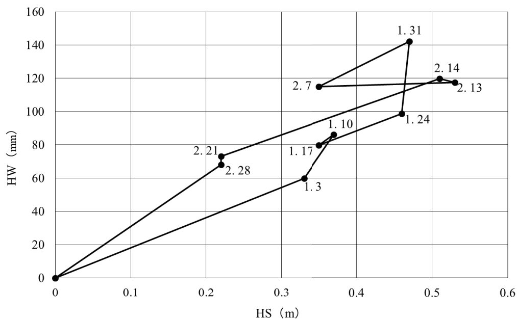
図5 雪氷防災研究センターにおける積雪深と積雪の相当水量の循環曲線(2018/19) Fig. 5 Relationship between the snow depth and the snow water equivalent at the SIRC (2018/19).
