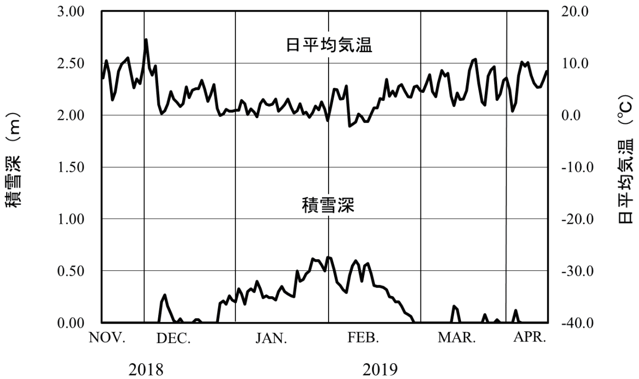
図 4.1 雪氷防災研究センターにおける積雪深および日平均気温の時間変化(2018/19) Fig. 4.1 Time series of the snow depth on the ground and daily mean air temperature at the SIRC (2018/19).
