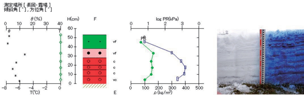
図 6.7 積雪断面観測値(長岡, 平成 31 年 2 月 13 日)
