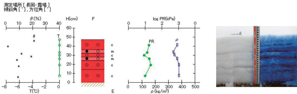
図 6.5 積雪断面観測値(長岡, 平成 31 年 1 月 31 日)
