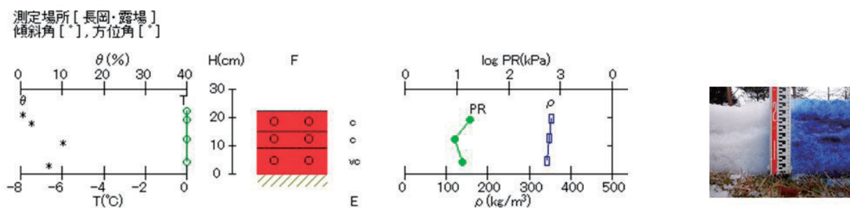
図 6.10 積雪断面観測値(長岡, 平成 31 年 2 月 28 日)
