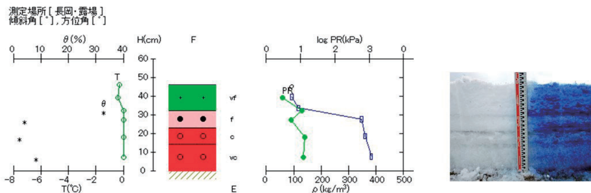
図 6.4 積雪断面観測値(長岡, 平成 31 年 1 月 24 日)
