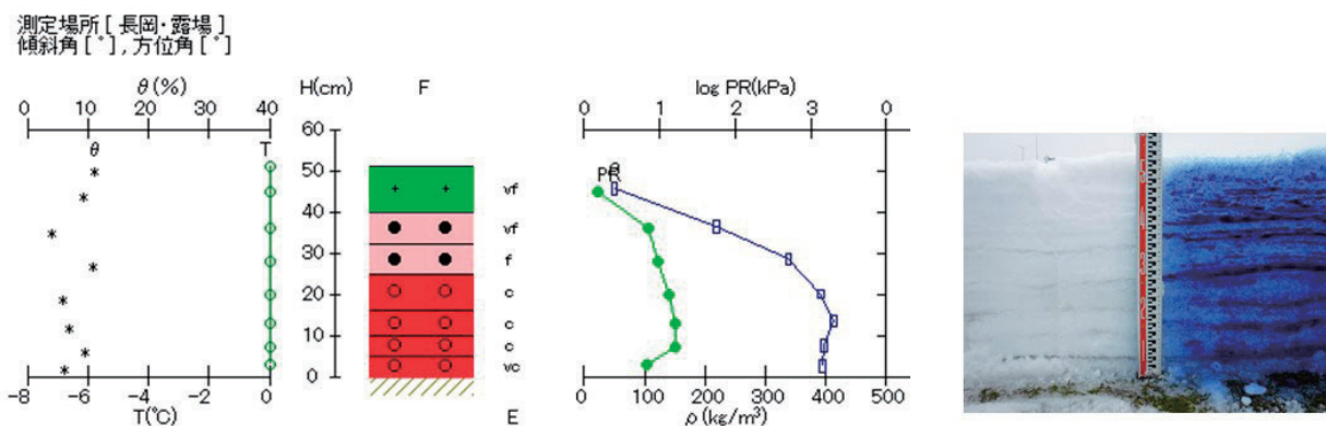
図 6.8 積雪断面観測値(長岡, 平成 31 年 2 月 14 日)
