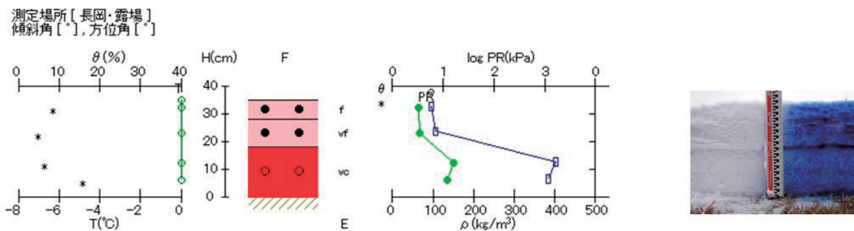
図 6.3 積雪断面観測値(長岡, 平成 31 年 1 月 17 日)
