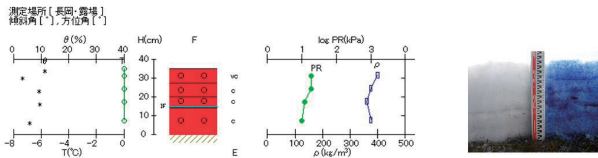
図 6.6 積雪断面観測値(長岡, 平成 31 年 2 月 7 日)
