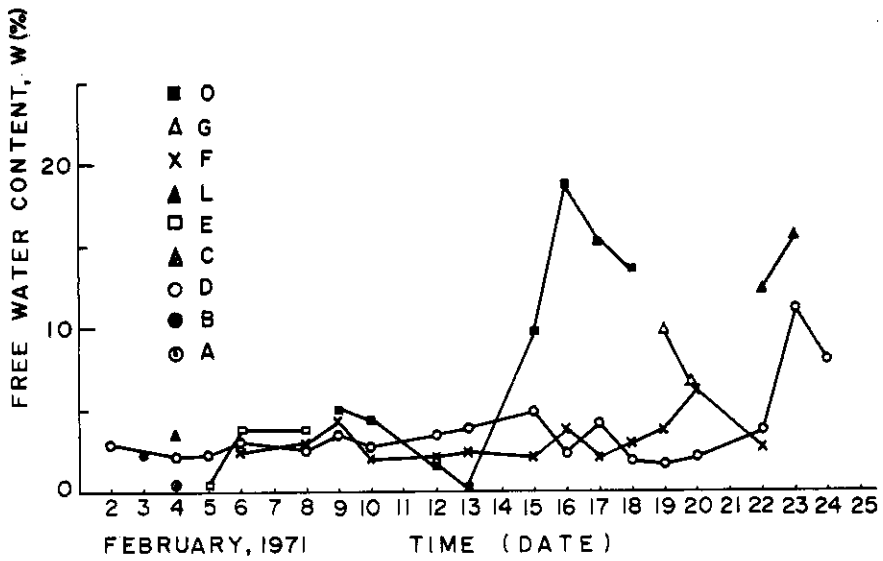
図 4 含水率の日変化
