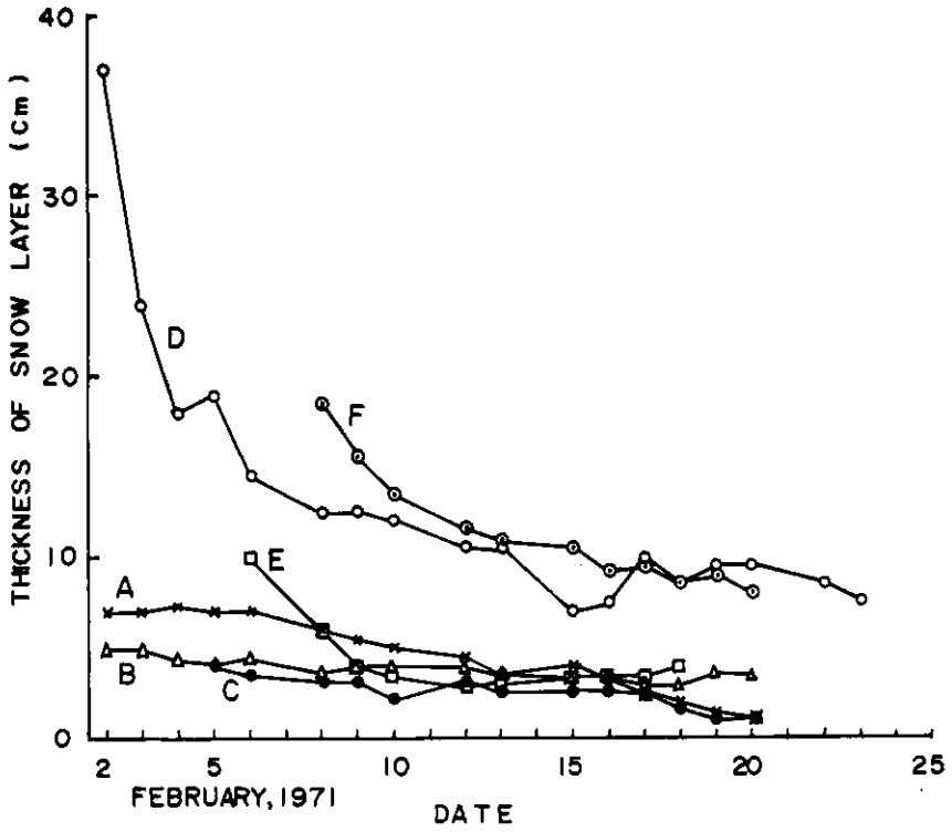
図 5 各積雪層の厚さの日変化
