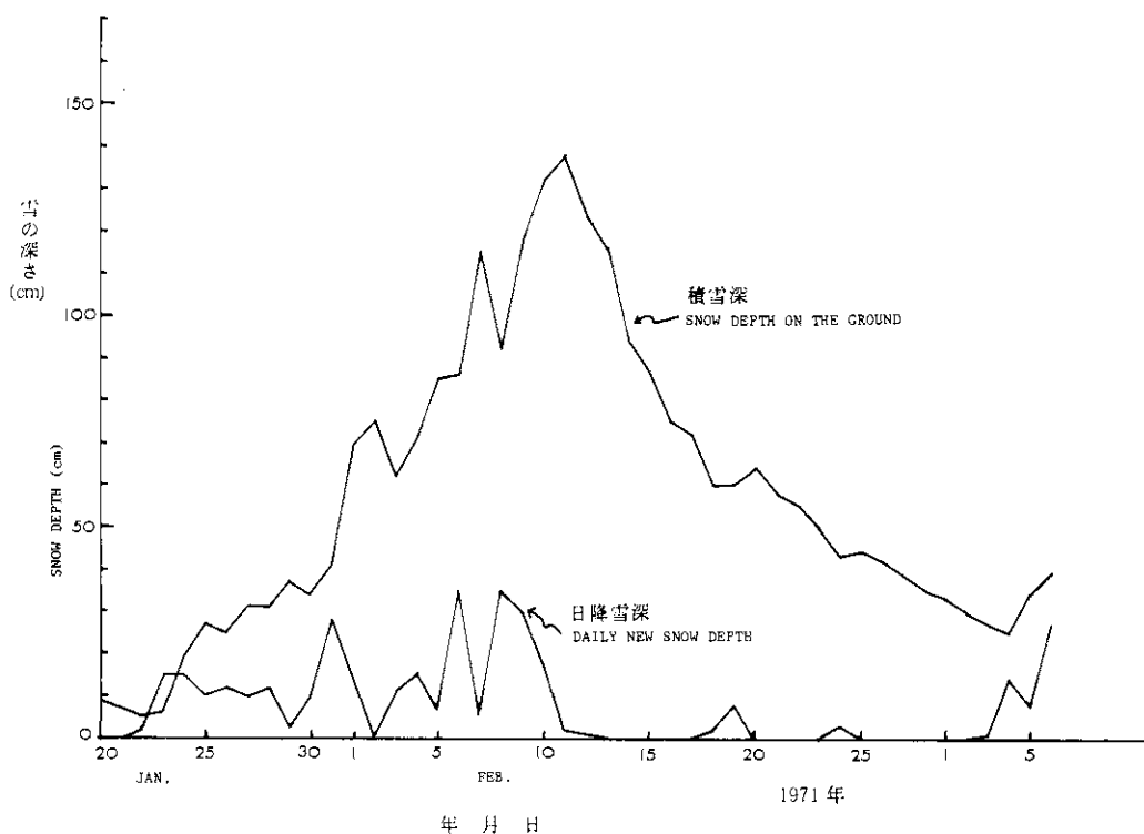
図 9 1971 年長岡における積雪深および日降雪深の変化
