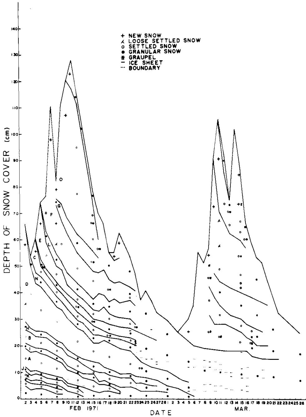
図 1 積雪深ならびに各成層構造の日変化 (図中のアルファベットは各層に与えた名前である)
