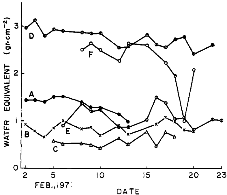
図3 各積雪層ごとの単位面積当りの質量の定常性 (ABCは各層名、以下同じ)
