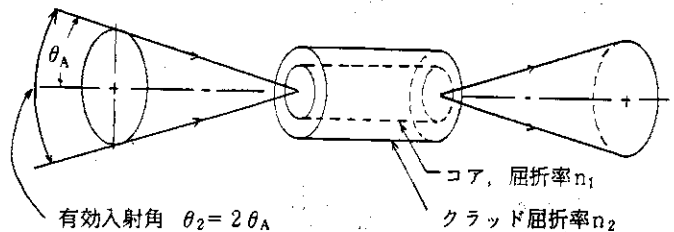
図 1.8 開口数 NA と有効入射角
