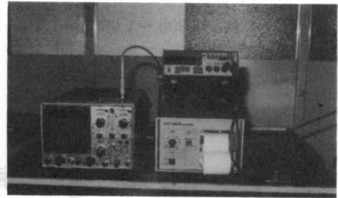
写真 3.3 測定系(右よりフォトセンサアンプ, デジタル電圧計およびレコーダ, オシロスコープ)
