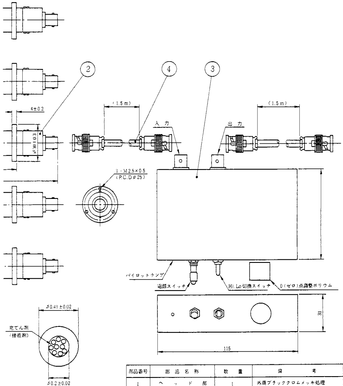
OF部(B)詳細図(80/1)
