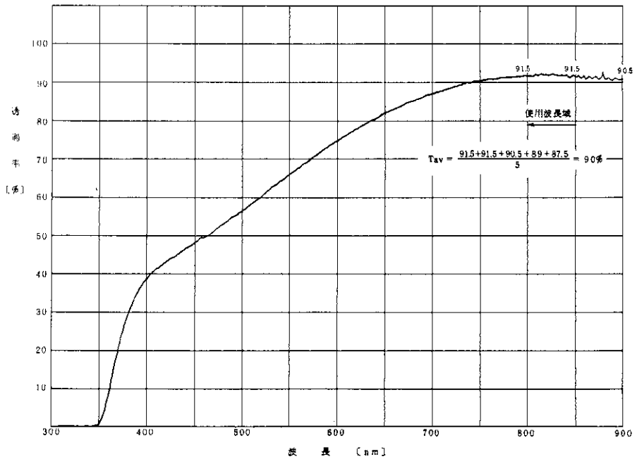
図 4.5 バンド 5, レンズ分光透過率 Fig. 4.5 Spectral transmissivity of lenses in light converging part, band 5.
